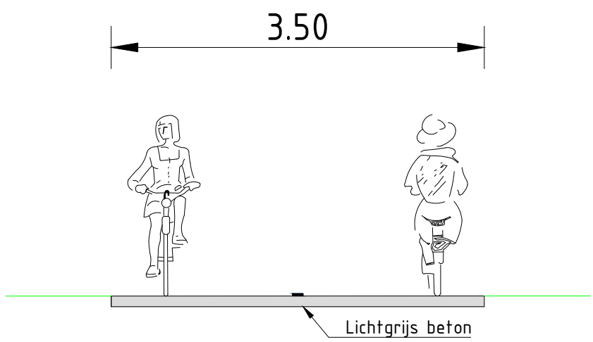
Dwarsprofiel Fietspad
