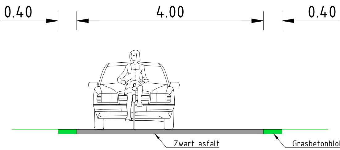
Dwarsprofiel Fietsstraat
