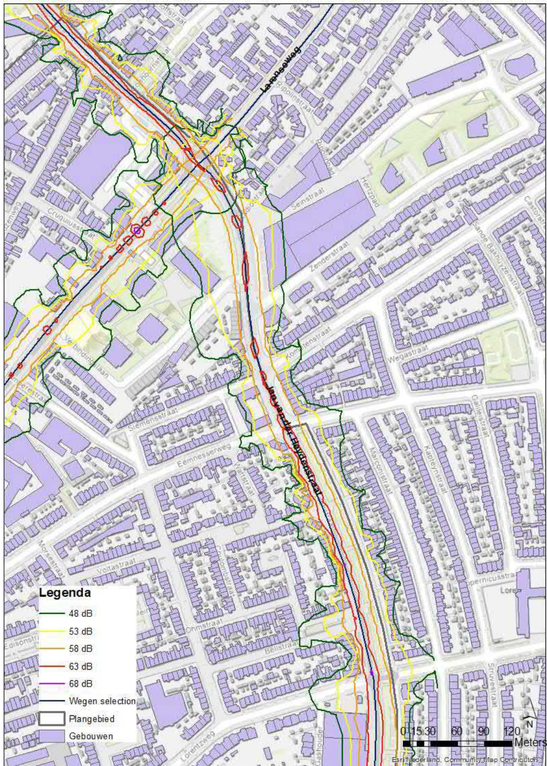
Figuur 4-3: Geluidcontouren van Jan van der Heijdenstraat en Larenseweg
