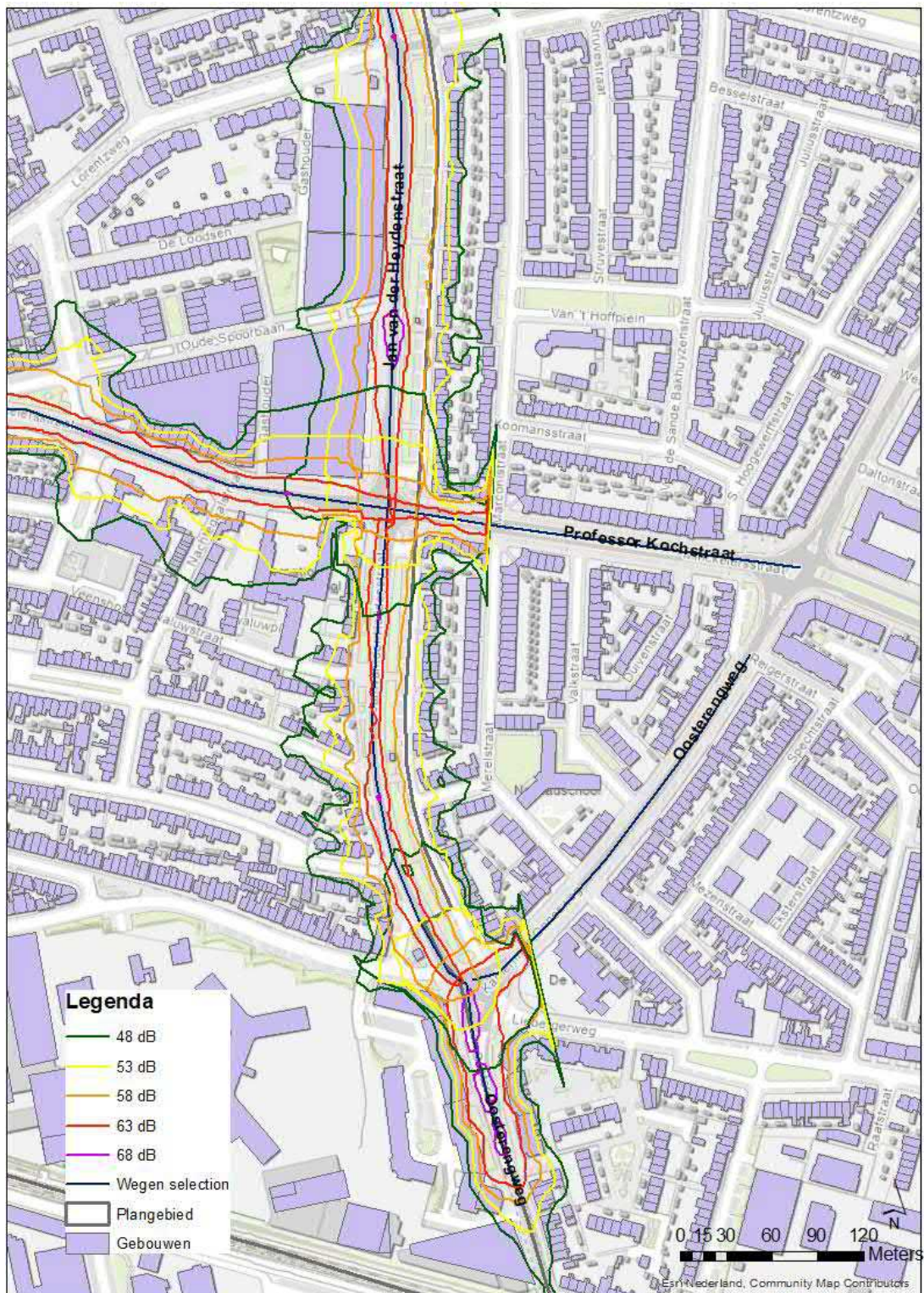
Figuur 4-1: Geluidcontouren van Oosterengweg en Jan van der Heijdenstraat
