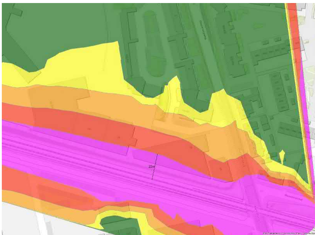
Figuur 4-6: Open veld contour railverkeerslawaai
