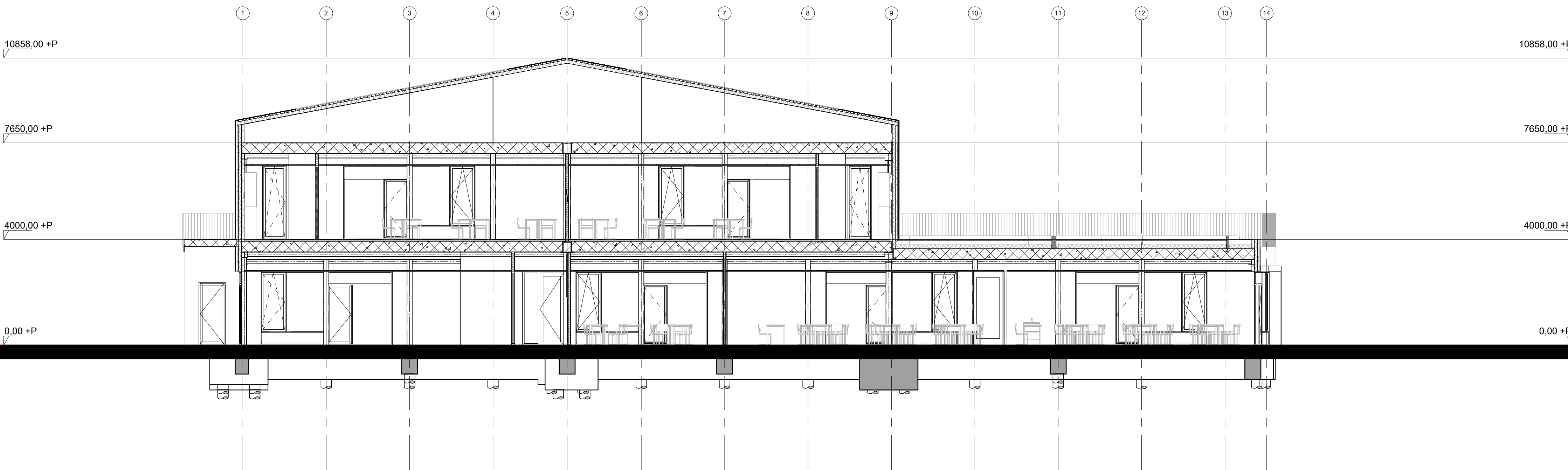
Doorsnede B-B
