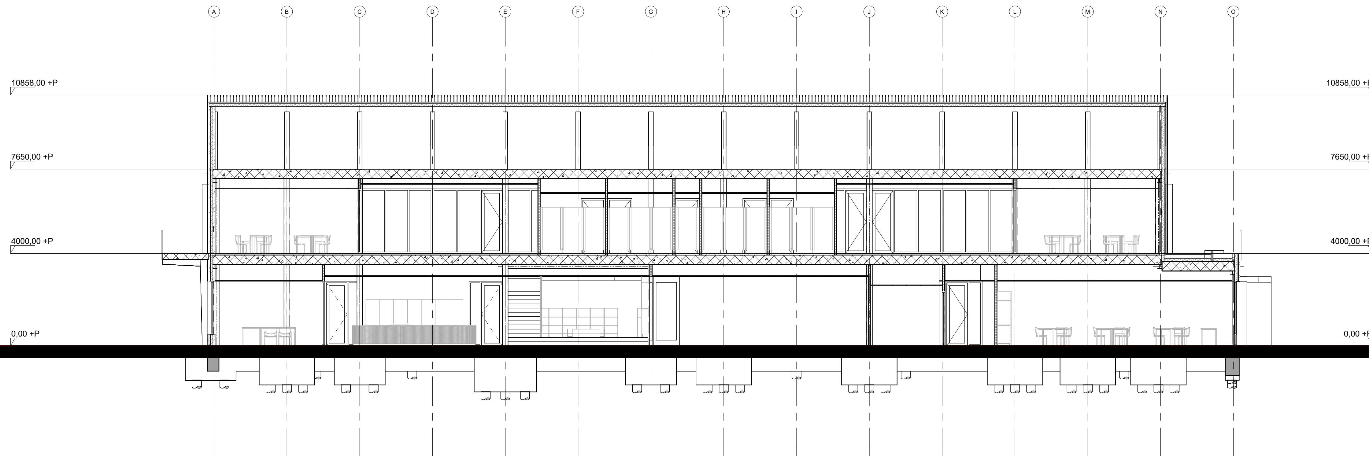
Doorsnede A-A
