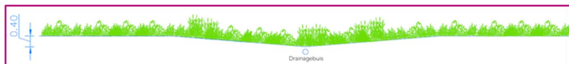
Figuur 3.12. Doorsnede wadi (bron: Stedenbouwkundig plan)
