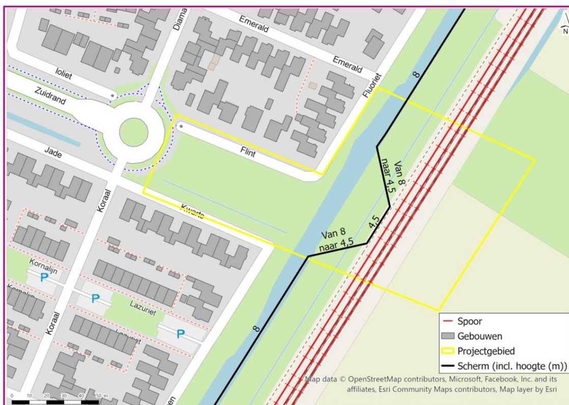
Figuur 2.13. Ontwerp geluidscherm Zuidrandtunnel variant 1
