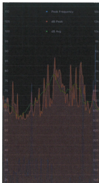
opnamen DBA meter zijgevel Kremselen 11a tijdens activiteit chippen
