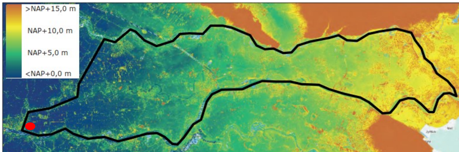
Figuur 3.6 Hoogteligging gebied Dijkkring 43, met aanduiding Gorinchem (rode stip) (VNK2, 2014)
