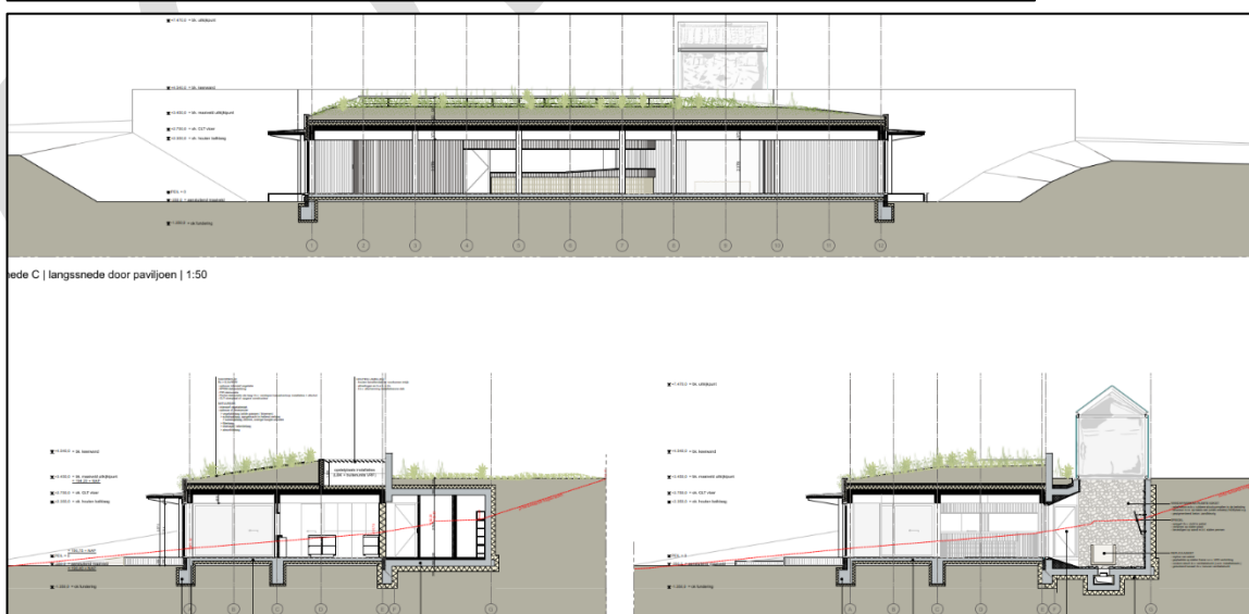
Aanzichten (links) en doorsneden (beneden)
