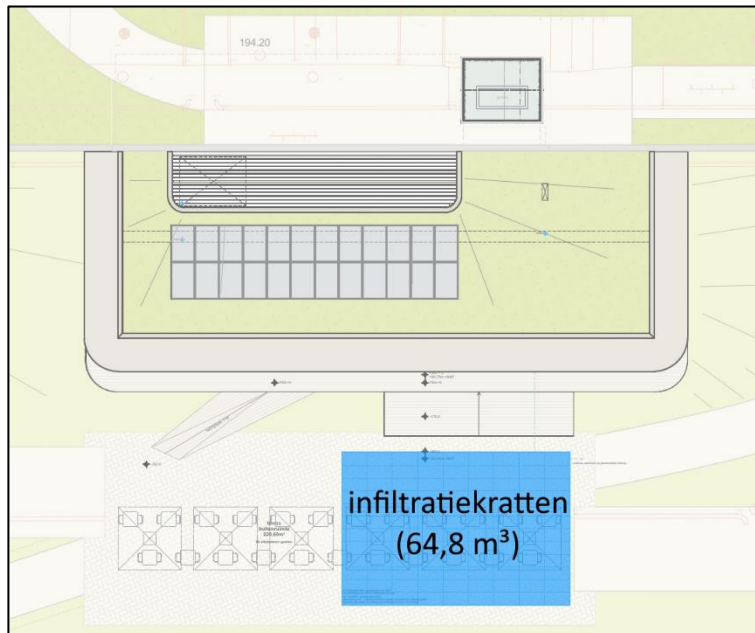
Situatietekening infiltratiekratten
