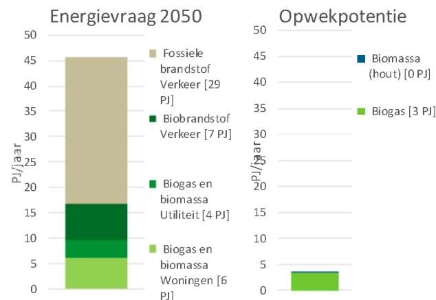
Figuur 9 Vraag en opwekpotentie van (bio)brandstoffen in 2050
