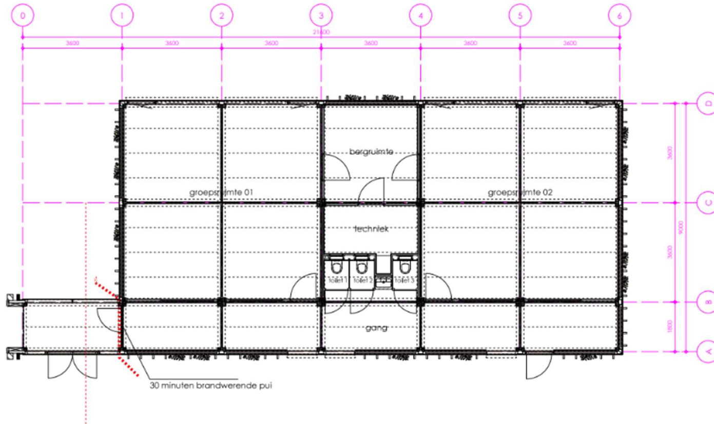
plattegrond uitbreiding
