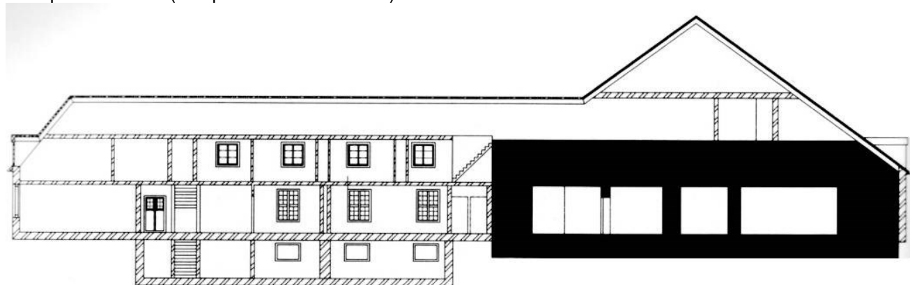
Doorsnee door het complex (naar RCE)
