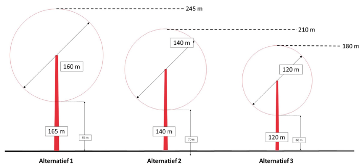
Figuur 1: Gegevens van de drie MER-alternatieven voor Windpark Beuningen.
