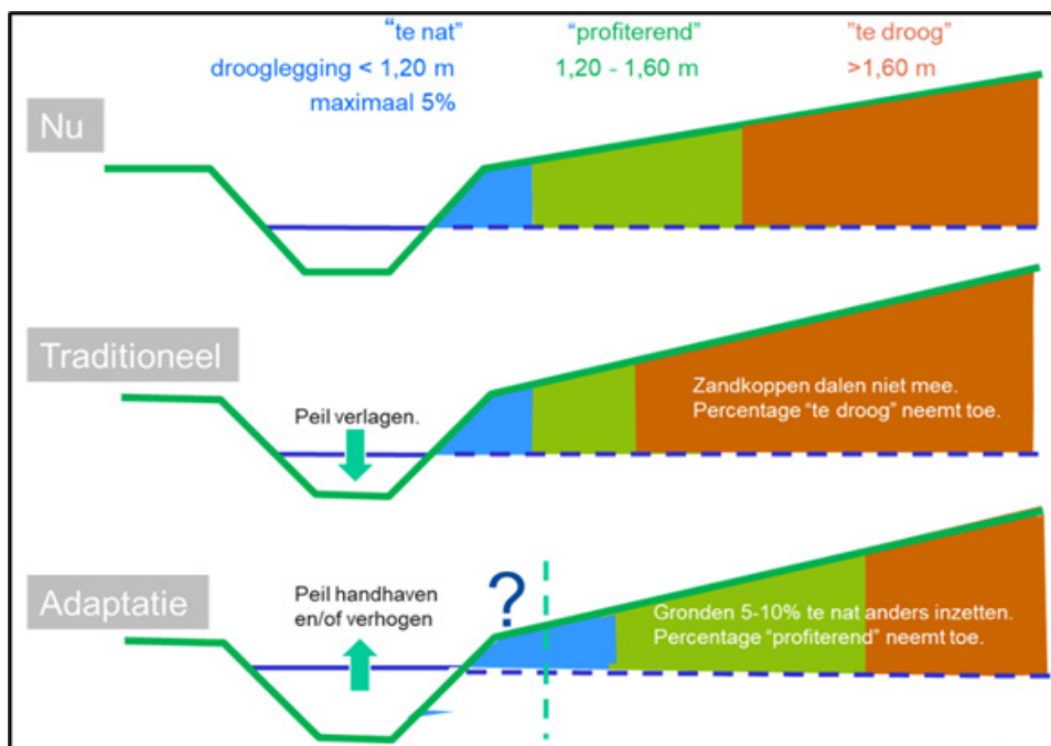
Afbeelding 22 uitleg peilbeheer
