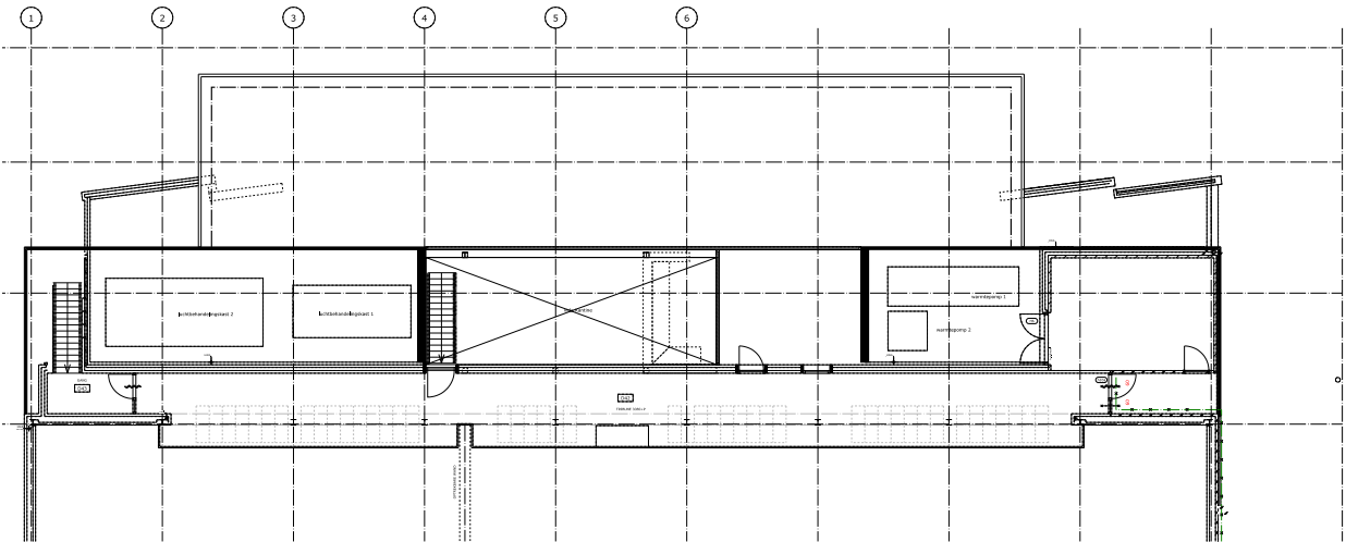
VERDIEPING
