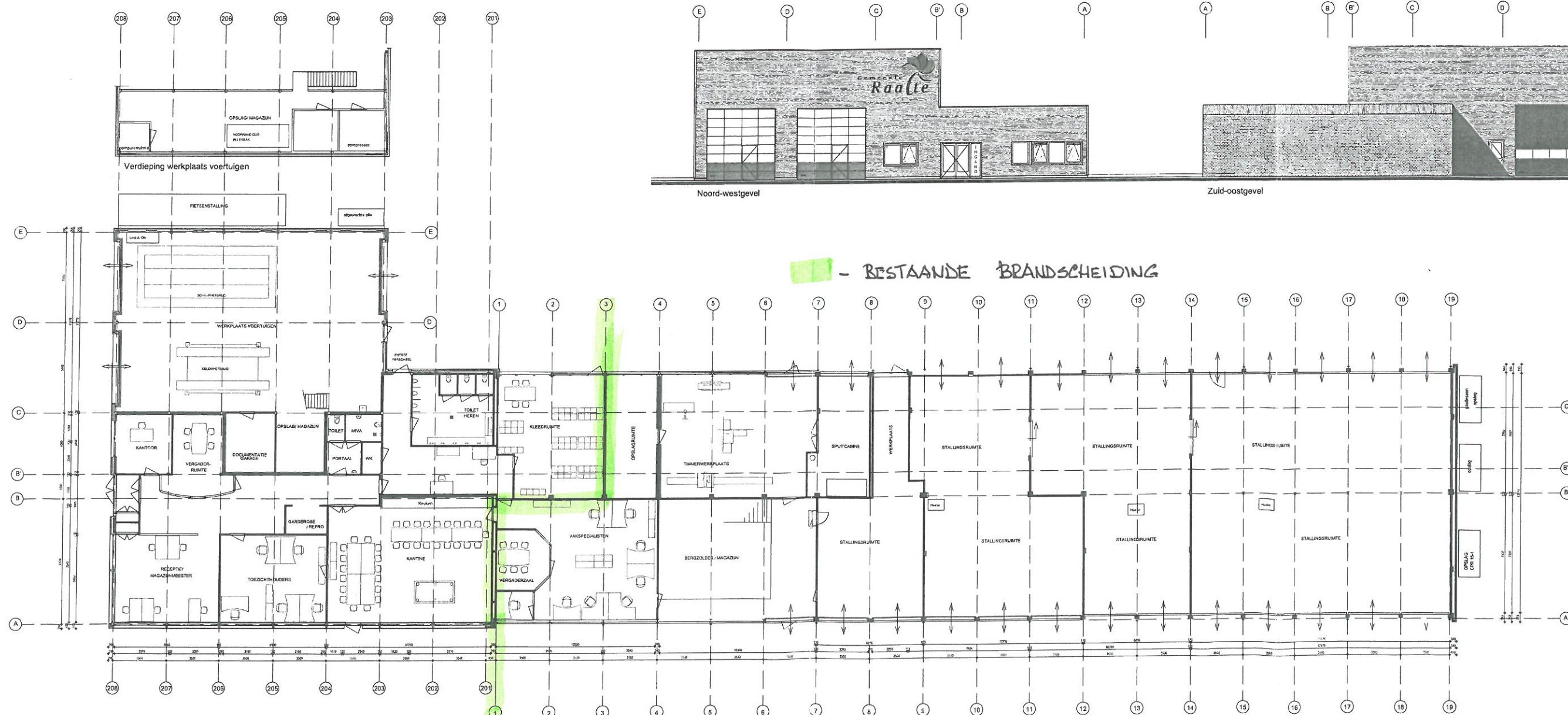
Begane grond - bestaand
