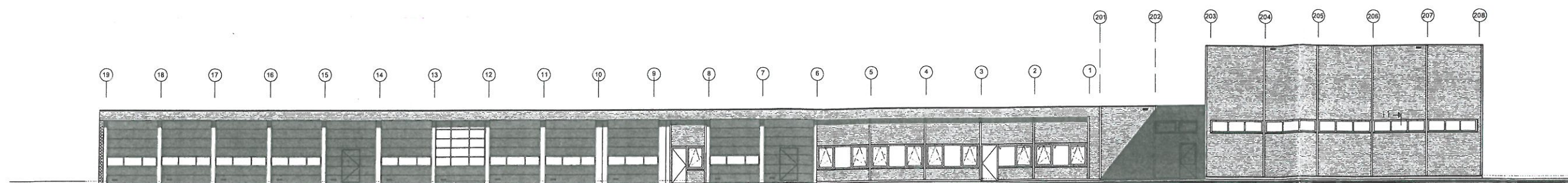
Noord-oostgevel
