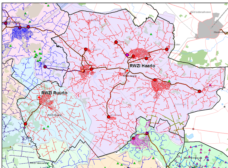
Figuur 2. Overzichtskartaal afvalwaterketen gemeente Berkelland. De rode lijnen geven de gemeentelijke riolering weer, de bruine lijnen de transportleidingen naar de RWZI's in Ruurlo en Haarlo.
