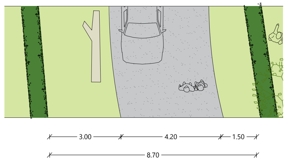
Profiel asfalt rijbaan éénrichting, deelgebied west (1:100)
