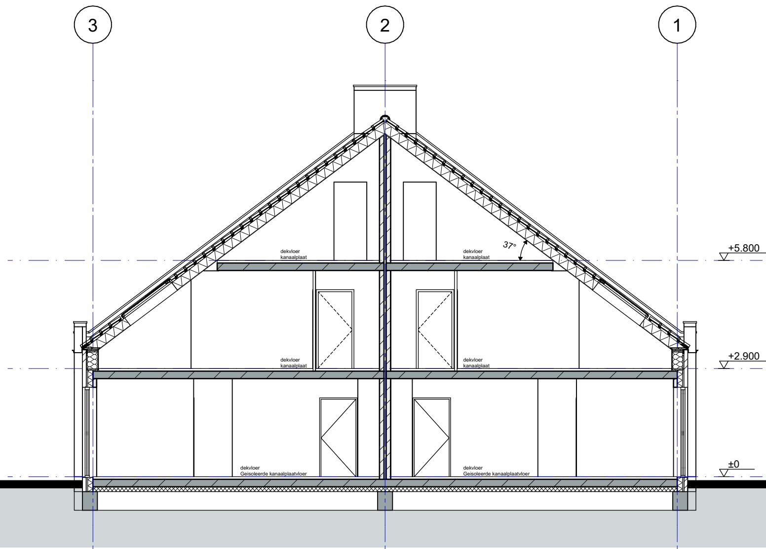
Doorsnede B-B
