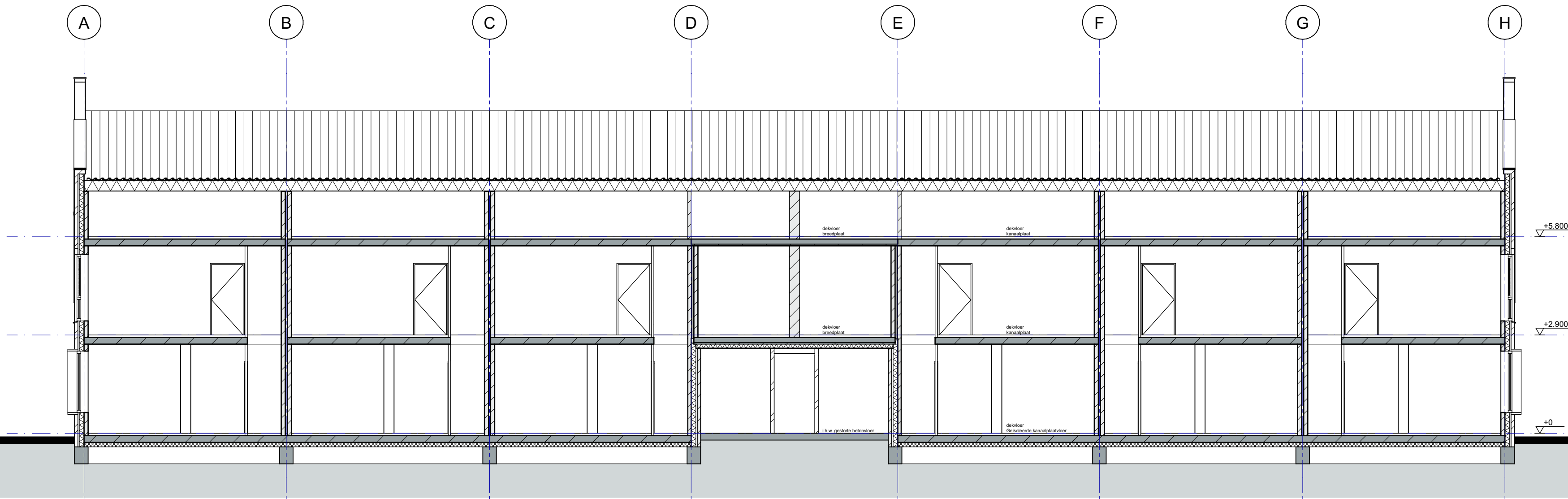
Doorsnede A-A
