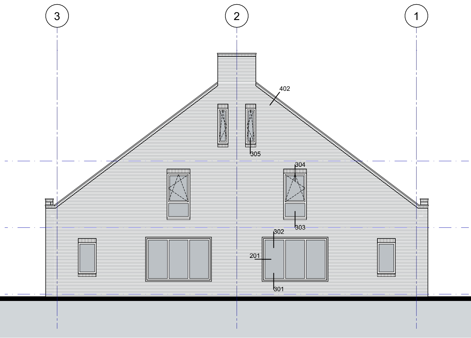
Noordgevel
