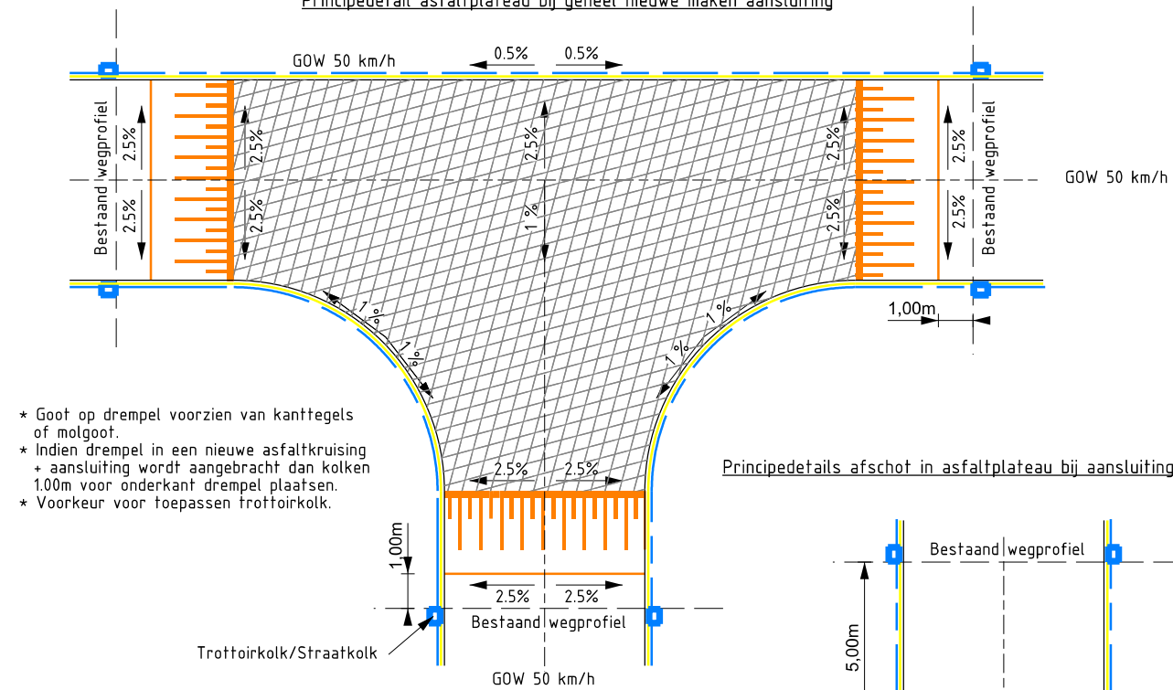
Principedetail asfaltplateau bij geheel nieuwe maken aansluiting
