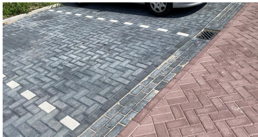
Figuur 11, haaks parkeervak betonstraatsteen antraciet, elleboogverband, markering ingestraat
