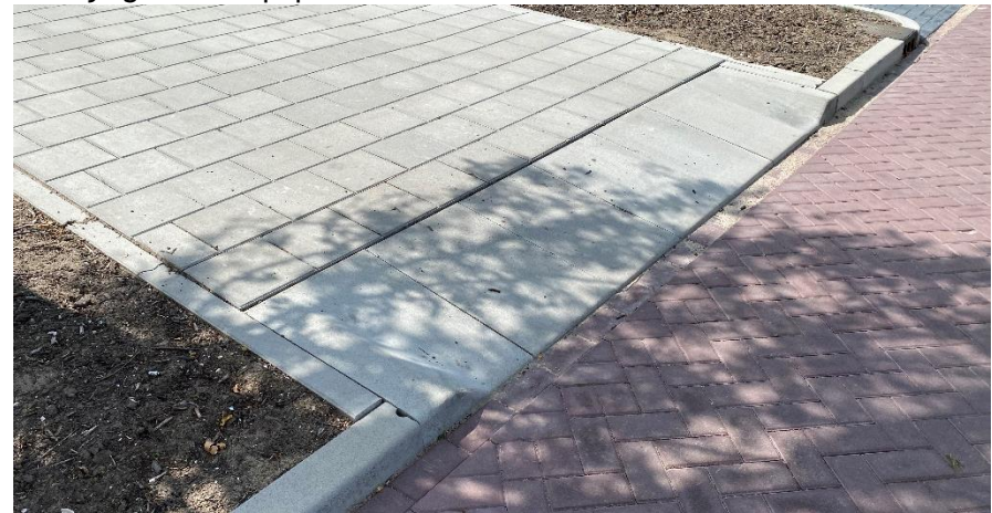
Figuur 8 inritconstructie. Locatie: Balkweiterhoek Zwaagdijk-West
