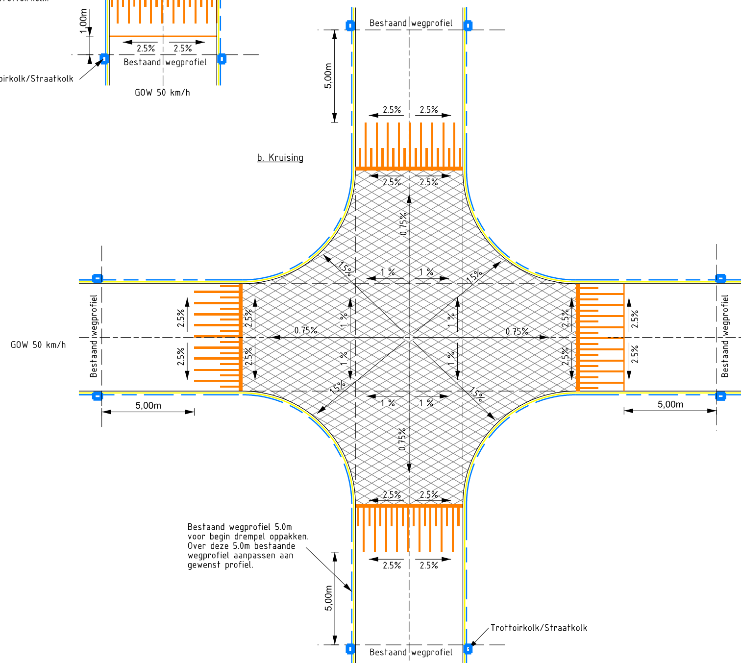
Principedetails afschot in asfaltplateau bij aansluiting in asfaltbestaand
