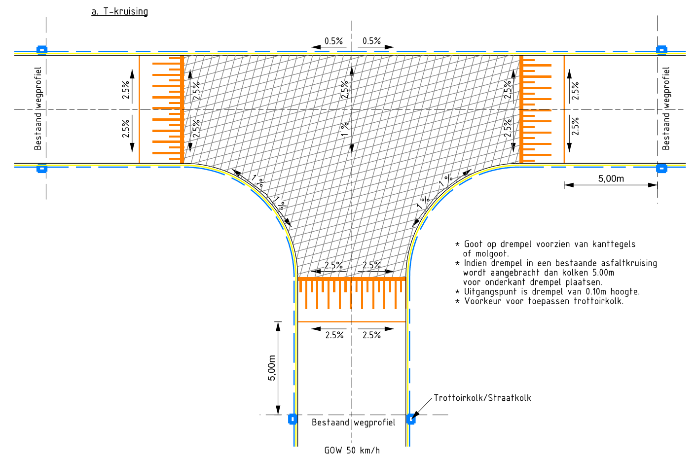
Principedetails afschot in asfaltplateau bij aansluiting in asfaltbestaand
