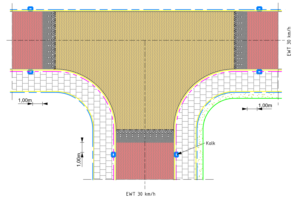
Principdetail plateau elementenverharding
