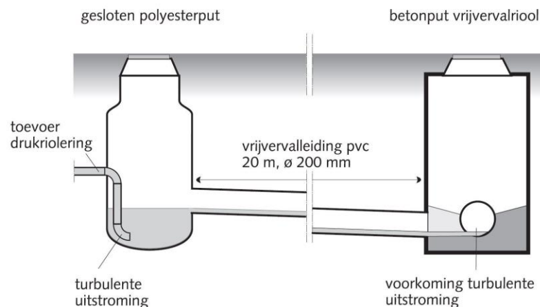
Figuur 17 principe aansluiting persleiding op vrijervalriool
