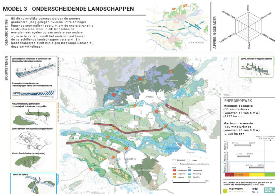
Afbeelding 4.13 Model 3 - Onderscheidende landschappen - indicatie alternatief landschap (H+N+S)
