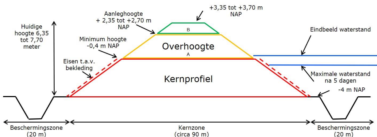
Figuur 3. Schematisatie profiel Knardijk met beschermingszone
