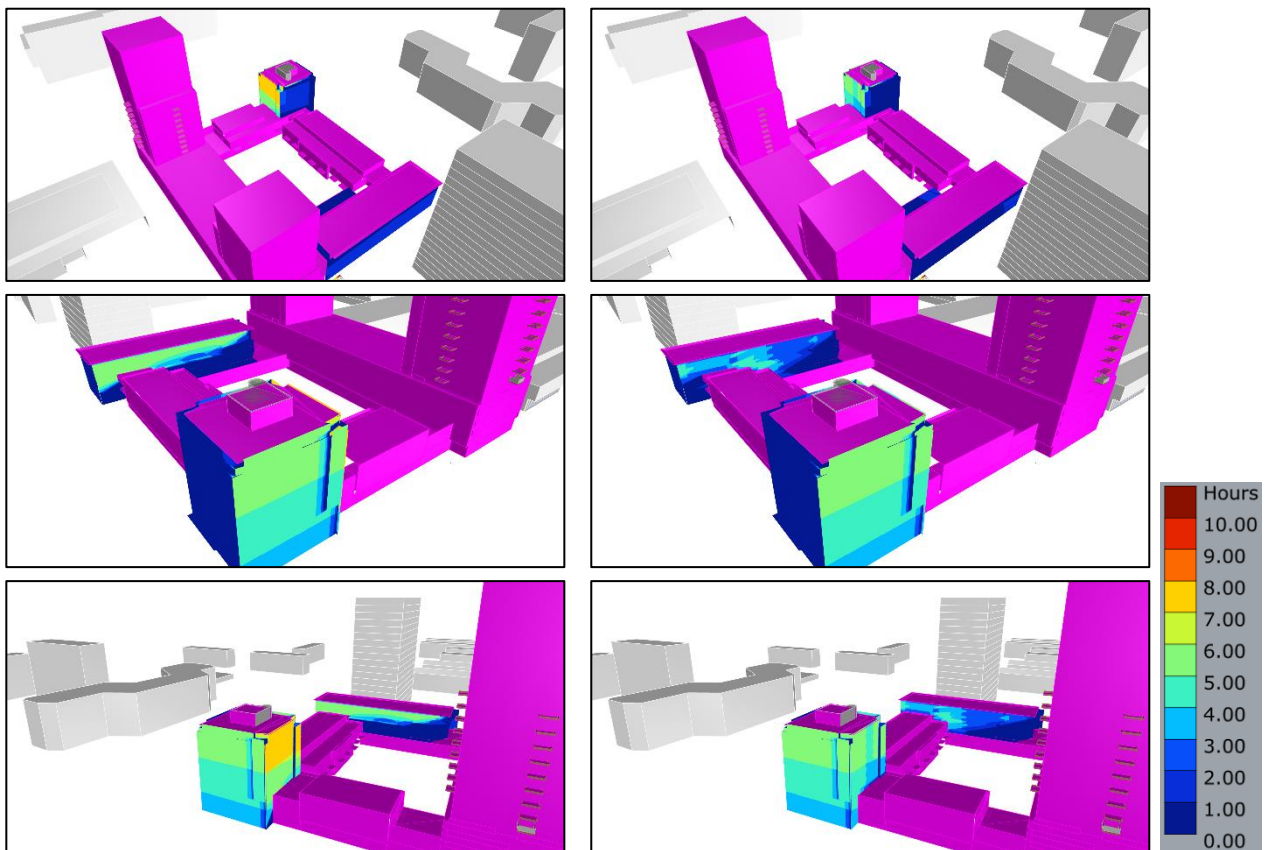
Figuur IV.2 Bezonningsduur bestaande situatie 21 december
