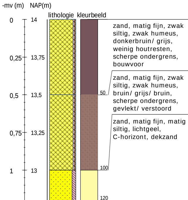
Boring 5 RD-coördinaten: 169790/467353
