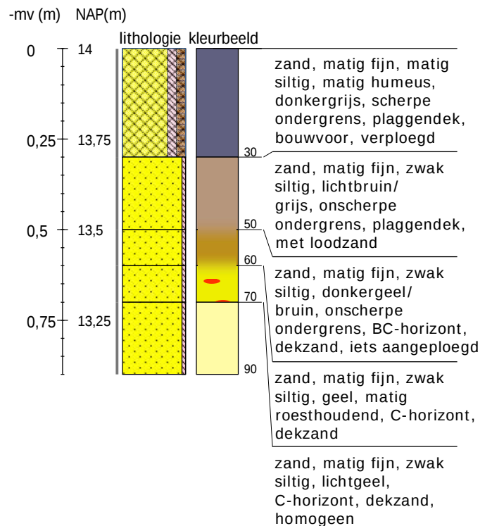
Boring 8 RD-coördinaten: 169800/467380
