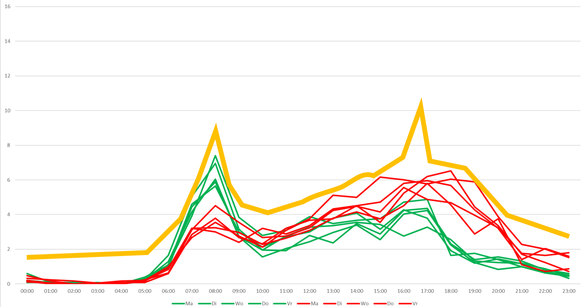
Fiets + auto Vredenburgweg OOST | week % van max capaciteit weg [1000] | Metingen Mobycon nov '21
