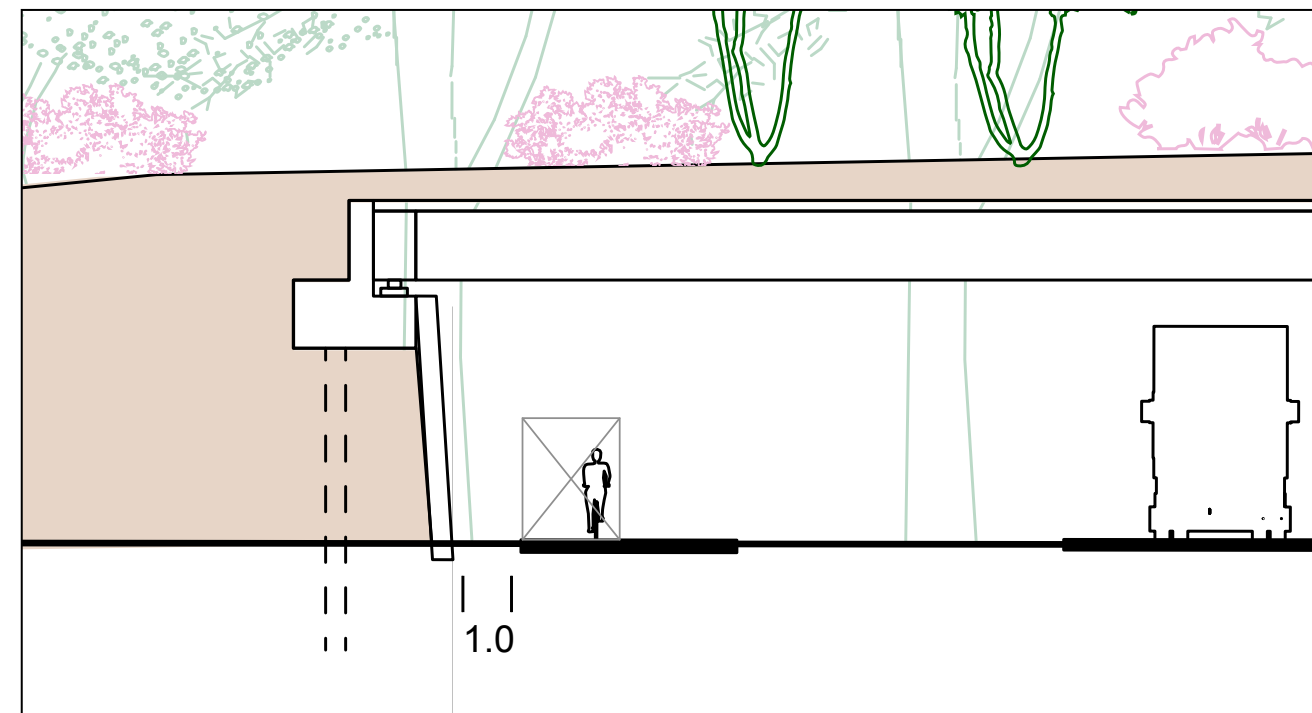
Landhoofd; oplegpunt
