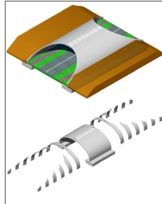
De randboogelementen
