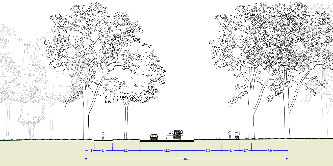
Doorsnede AA'
