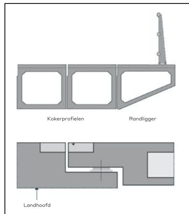
Kokerprofielen en oplegpunt
