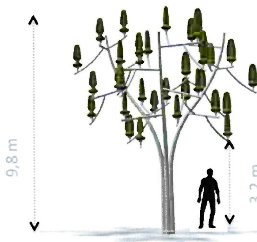
Afbeelding 2: Afmeting windtree
