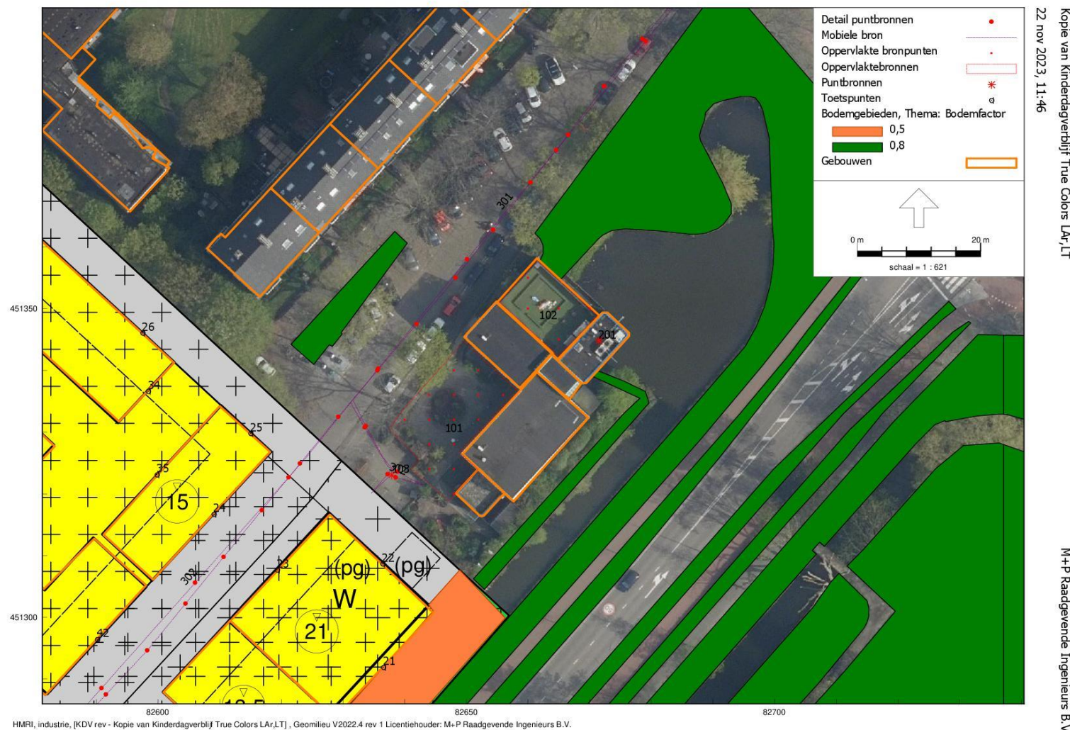
figuur 3 rekenmodel KDV, L_{Ar,LT} bronnen binnen de inrichting en indirecte hinder (bon 301 en 303), standaard bodemfactor = 0,2
