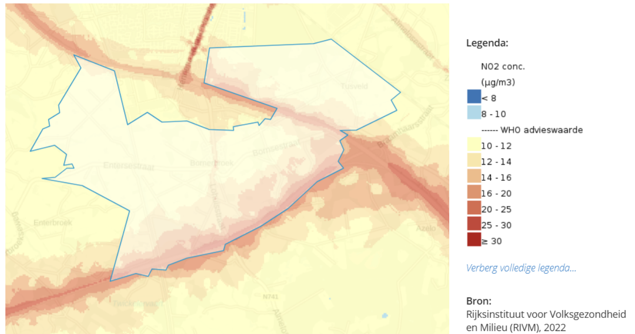
Figuur 3.13 - NO 2 -concentratie in Bornerbroek.
