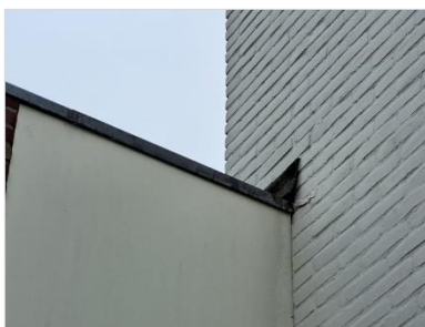
Figuur 4.5 Ruimte achter loshangende loodslab bij bebouwing 2.
