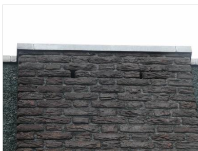
Figuur 4.7 Open stootvoegen bij bebouwing 4.
