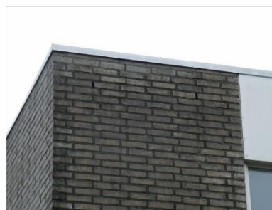
Figuur 4.9 Open stootvoegen bij bebouwing 6.
