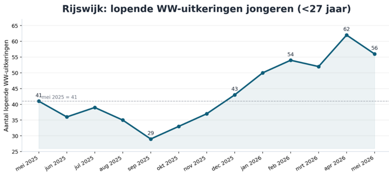
Figuur 1. Maandelijkse ontwikkeling lopende WW-uitkeringen jongeren in Rijswijk.
