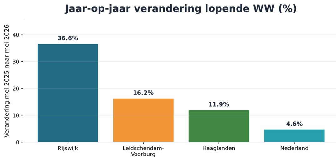
Figuur 4. Procentuele jaar-op-jaarverandering lopende WW-uitkeringen jongeren. Bron: UWV Dashboard WW-uitkeringen, export verwerkt 2 juli 2026.
