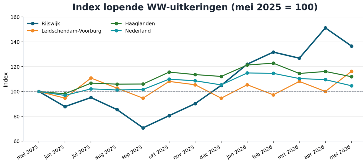
Figuur 3. Index lopende WW-uitkeringen jongeren, mei 2025 = 100. Bron: UWV Dashboard WW-uitkeringen, export verwerkt 2 juli 2026.
