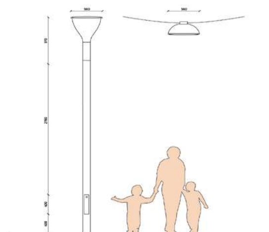
Q-impuls Lichtmast en hangarmatuur
