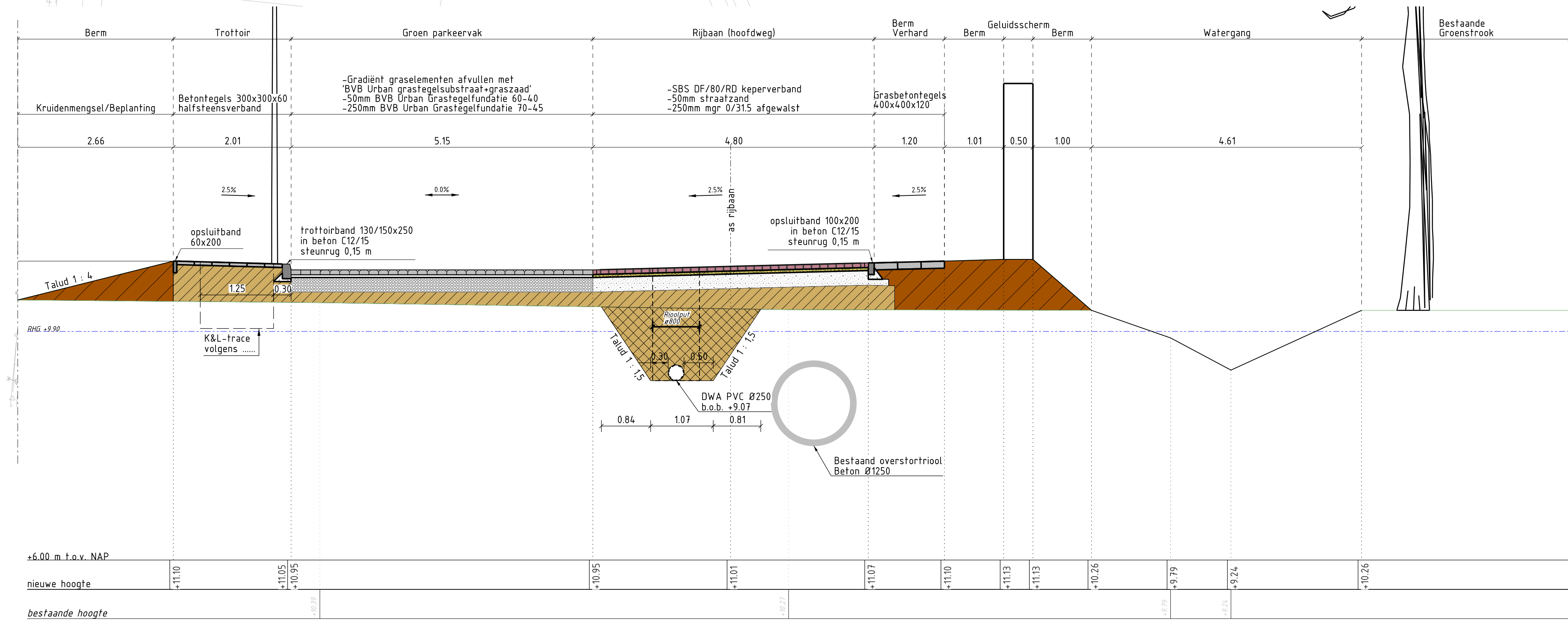
Dwarsprofiel 3
