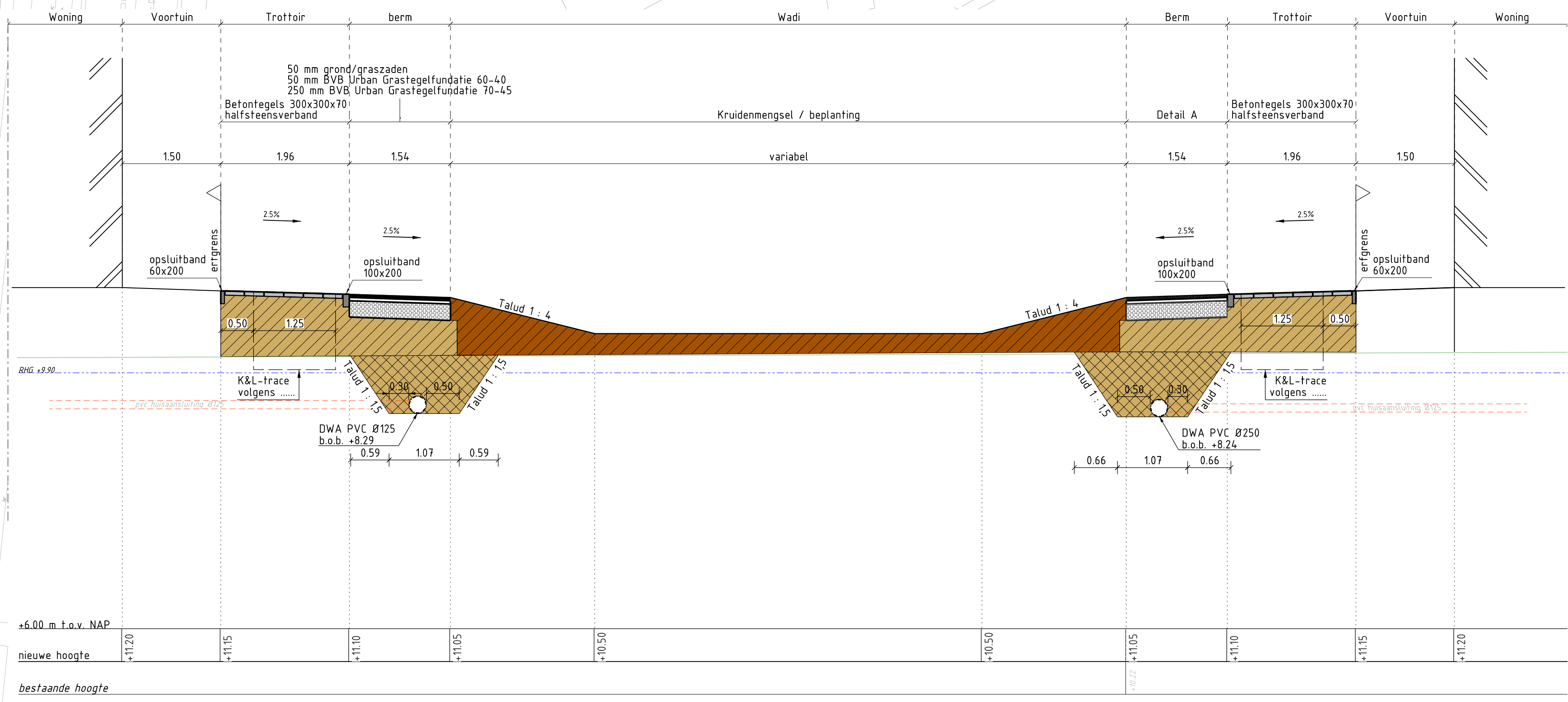
Dwarsprofiel 1
