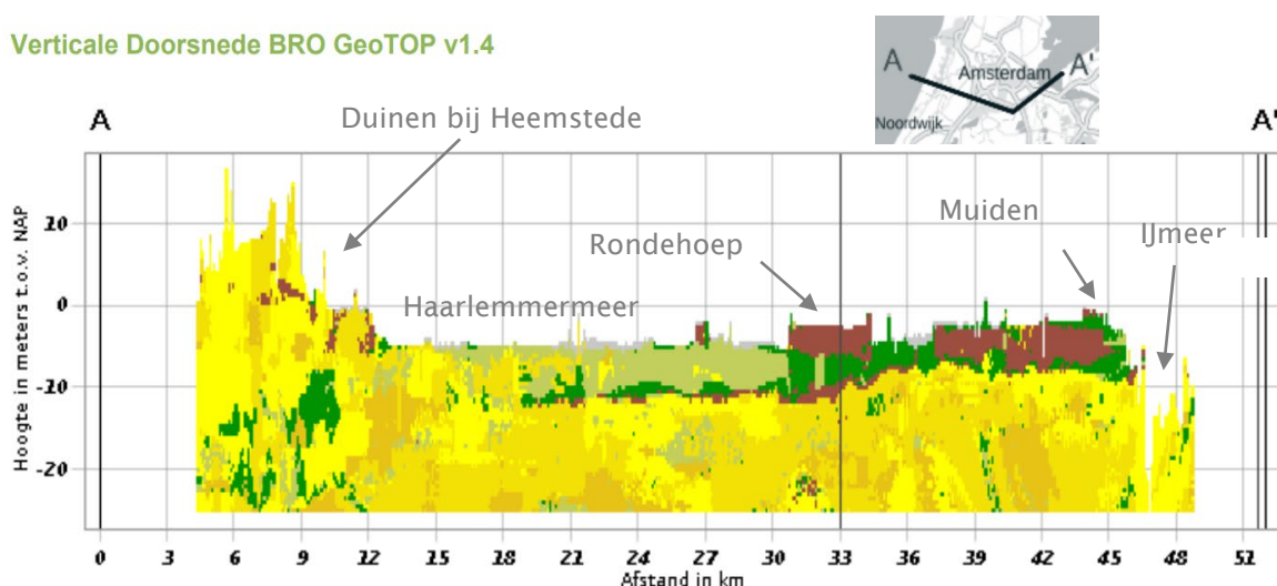
Figuur 6 dwarsdoorsnede
