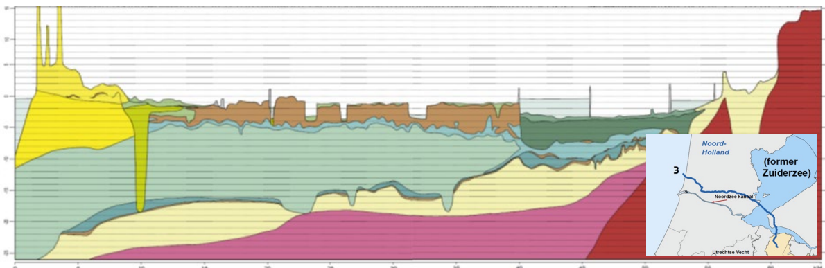
Figuur 5 Geologische dwarsdoorsnede van Laag Holland (bruin = veen, geel/paars = zand en groen/blauw = klei (Vos, 2015)
