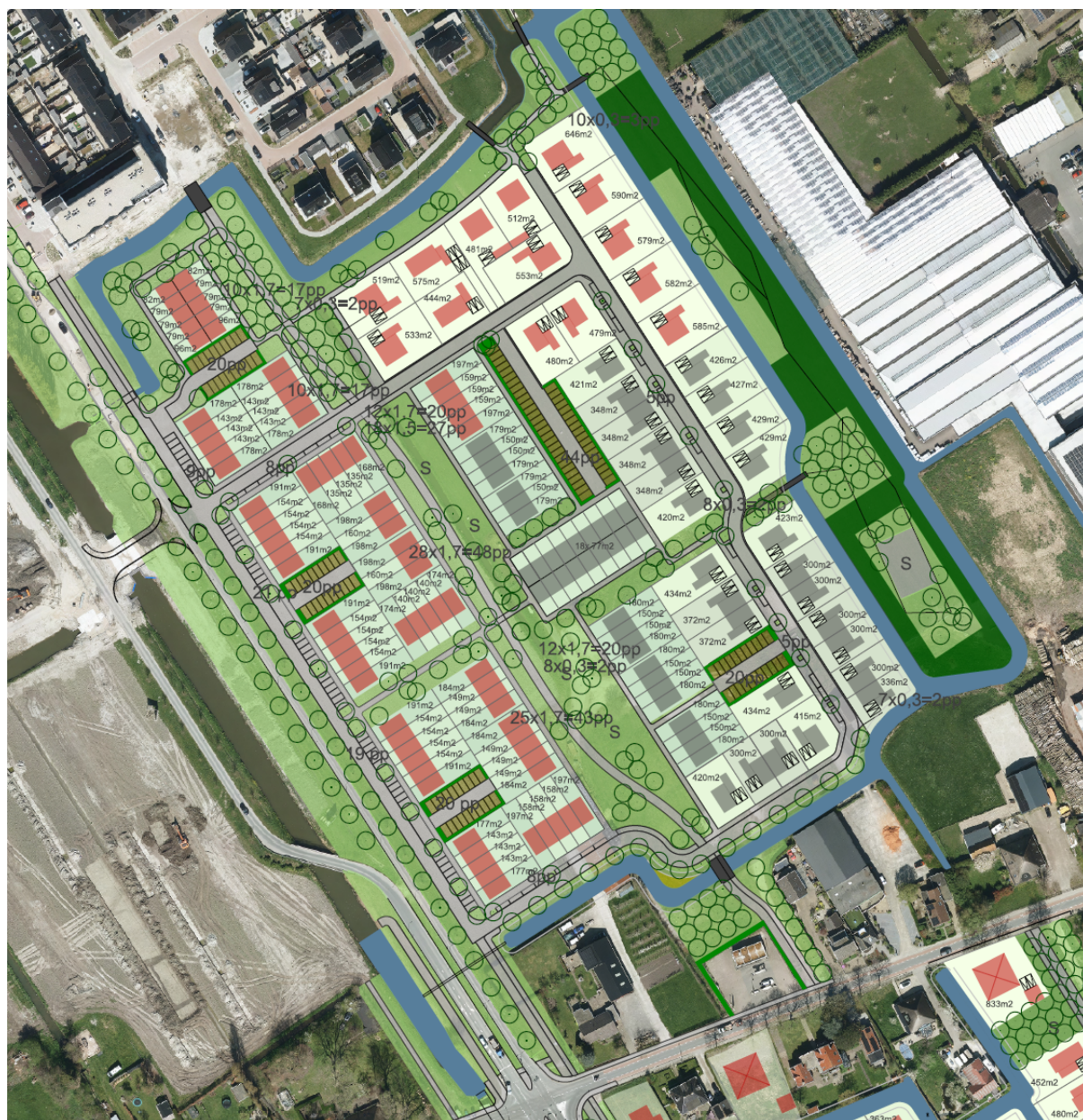
Figuur 2.2: Verkaveling
