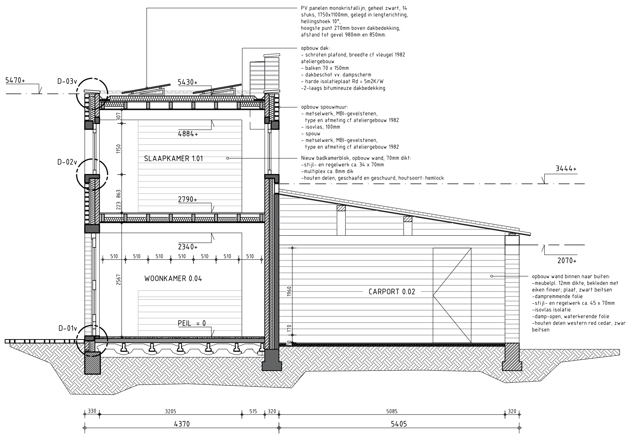
DOORSNEDE DD
