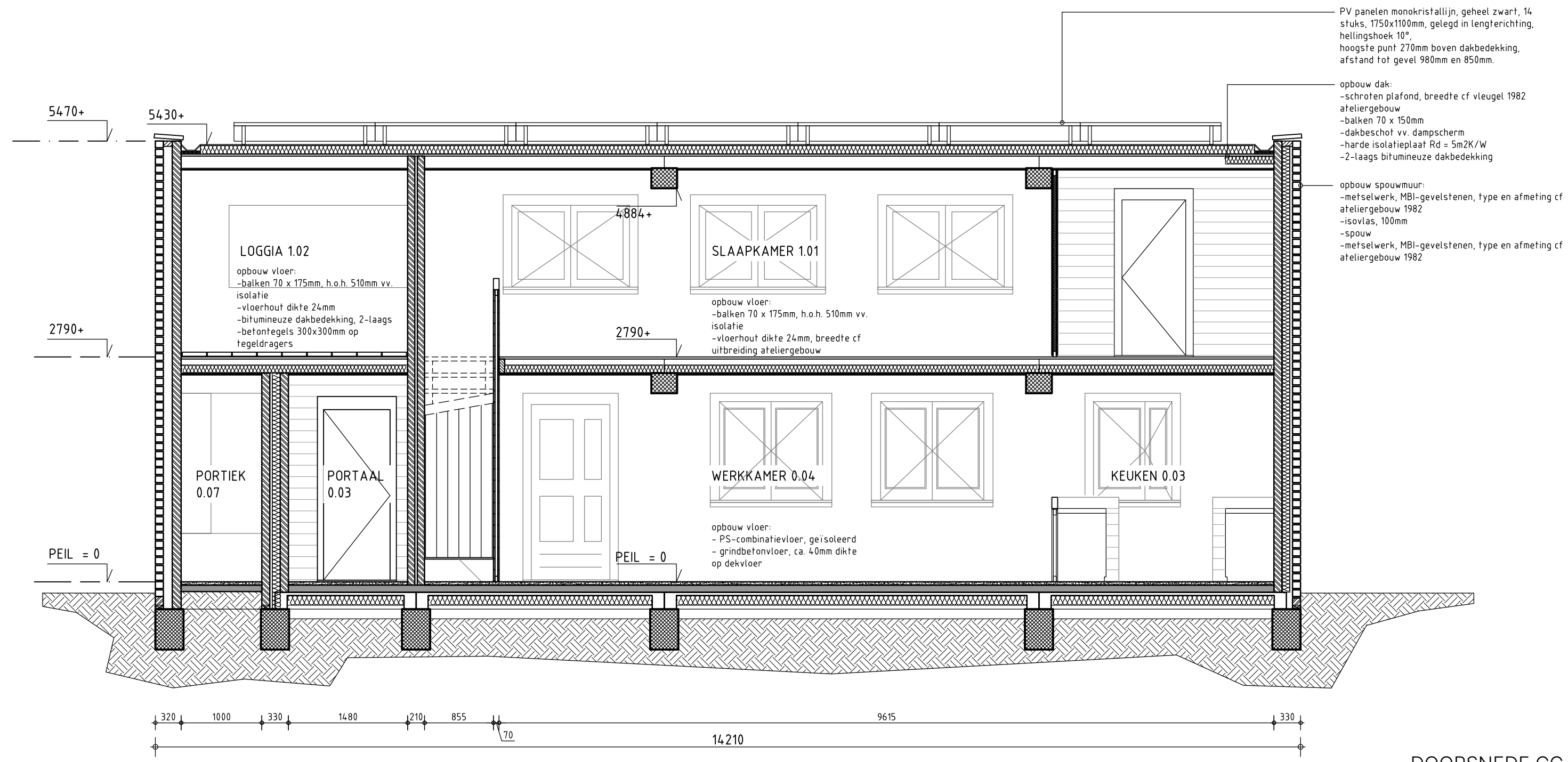
DOORSNEDE CC
