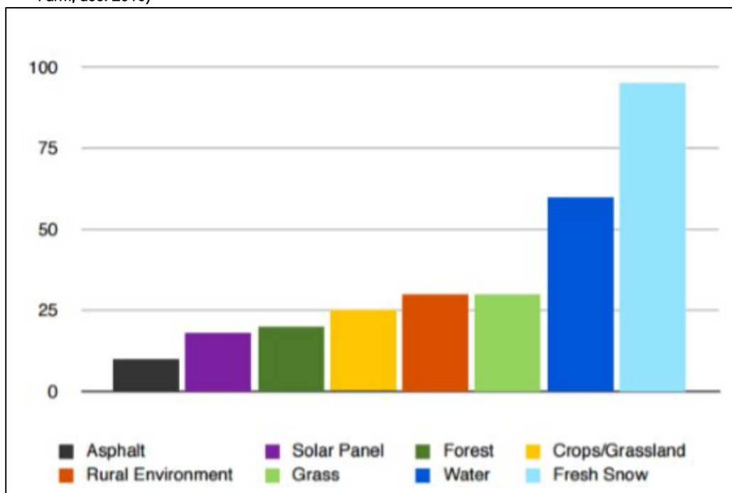
figuur 26. Lichtreflectie zonnepaneel en andere veel voorkomende materialen (bron: Visual Impact Assessment, VK, Capital Solar Farm, dec. 2010)
