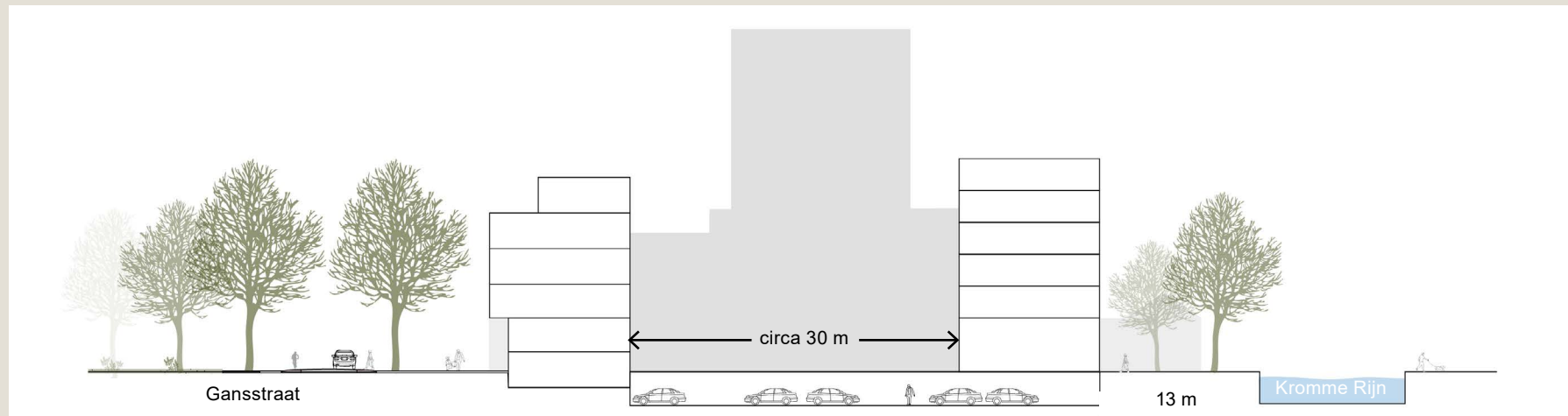
Dwarsdoorsnede 3: volledig verdiepte parkeeroplossing
