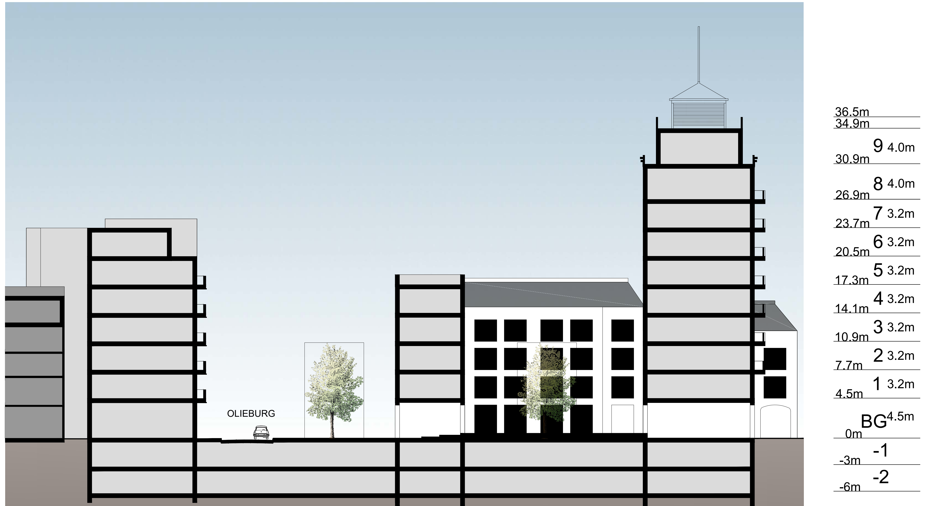
PRINCIPE DOORSNEDE 02
