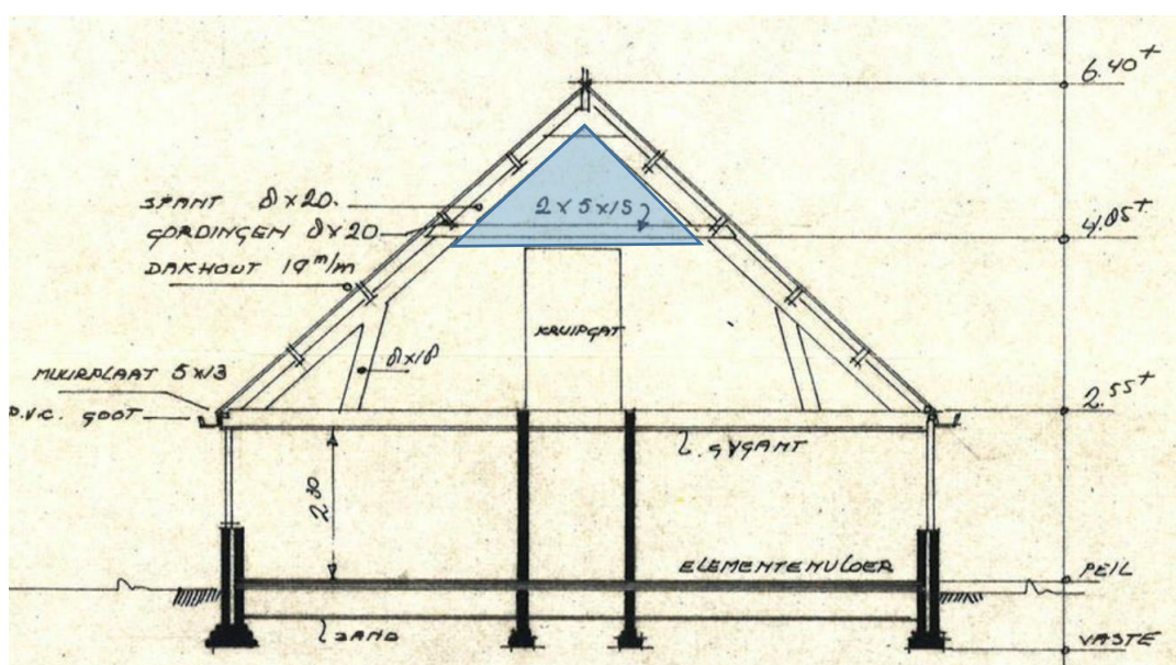
Figuur 20 Doorsnede van de oostzijde van de woning Achteromweg 3. Het af te timmeren deel is blauw gemaakt.
