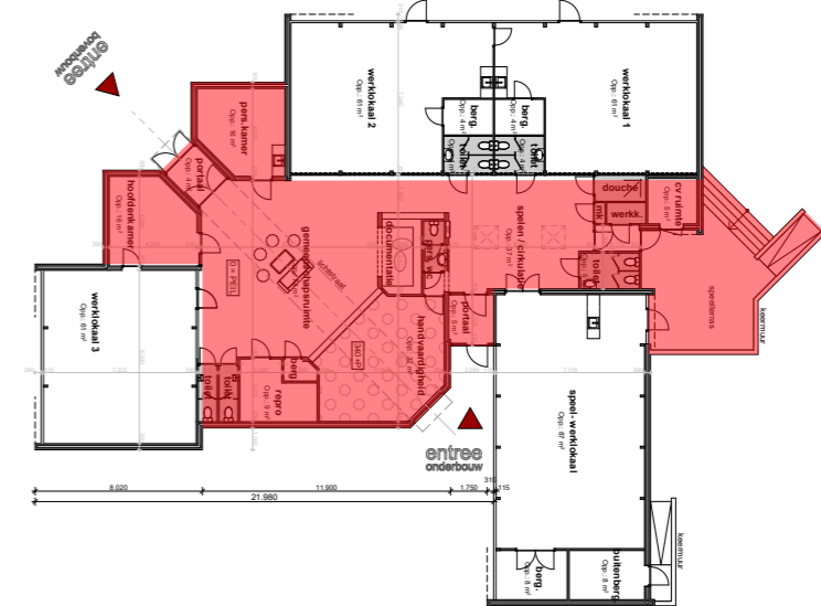
bestaande plattegrond met te slopen volume's
