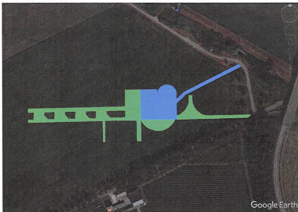
Turbine 1 – permanente en tijdelijke verhardingen
