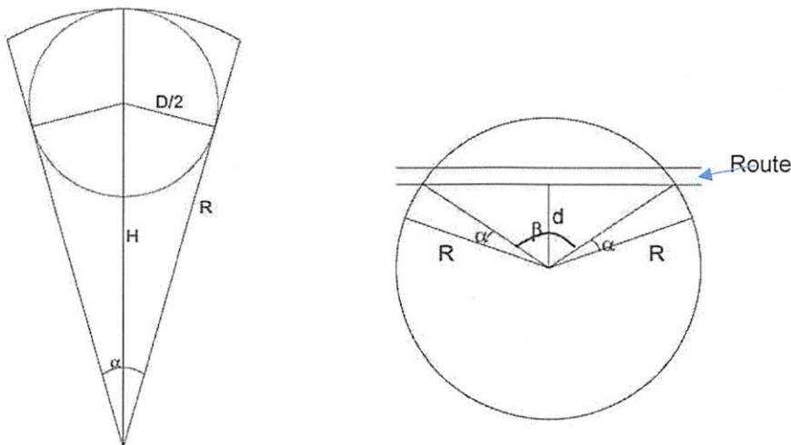
Maatvoering in vooraanzicht (links) en bovenaanzicht (rechts) van turbine en route
