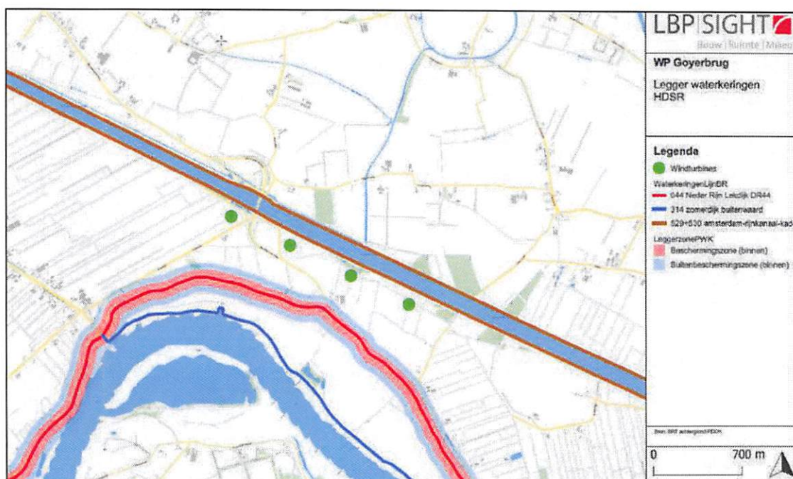
Figuur 4.20 Primaire waterkering ter plaatse van de Lekdijk
