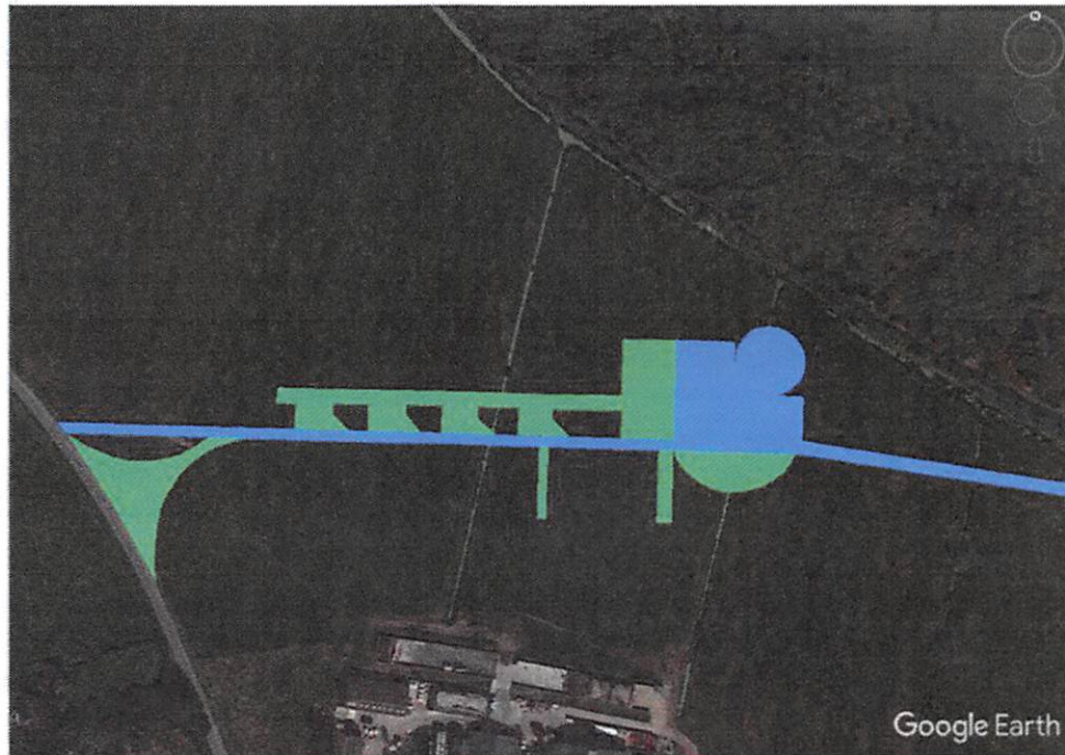
Turbine 3 – permanente en tijdelijke verhardingen
