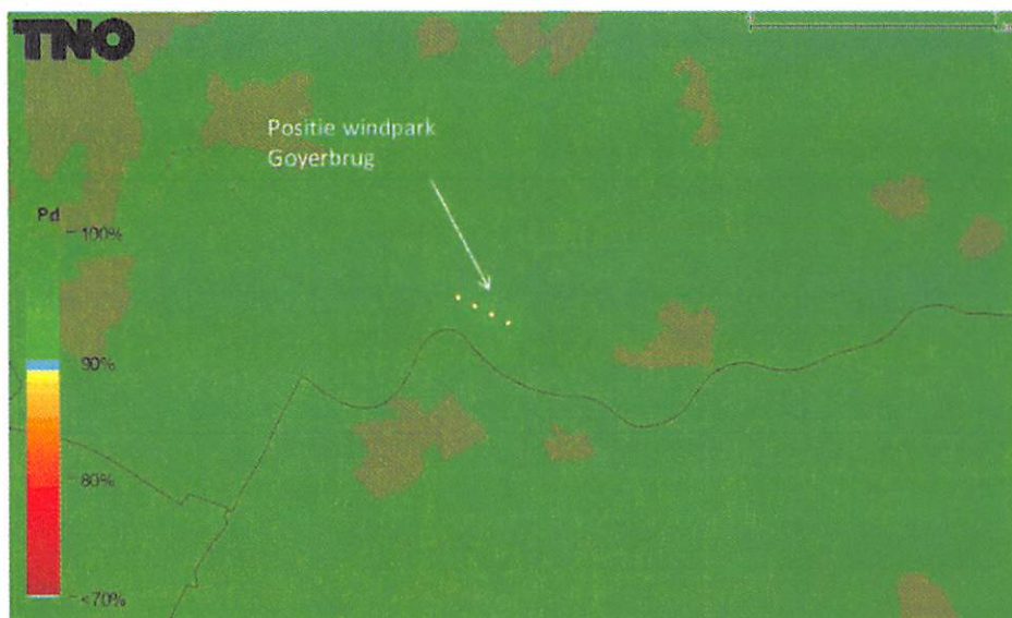
Figuur 6 Detectiekans van het primaire verkeersleidingsradarnetwerk op 1000 voet boven het bouwplan nadat deze is gerealiseerd. De locatie van de nieuwe windturbines is aangegeven met gele stippen.
