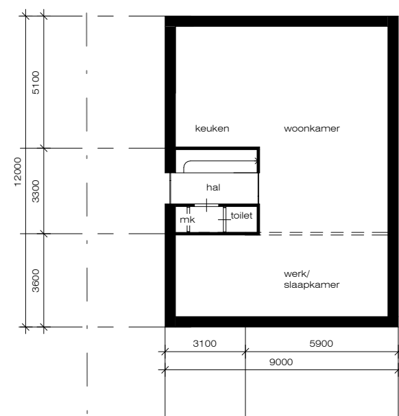
begane grond
