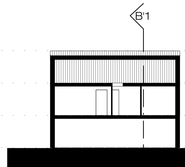
doorsnede A-A
