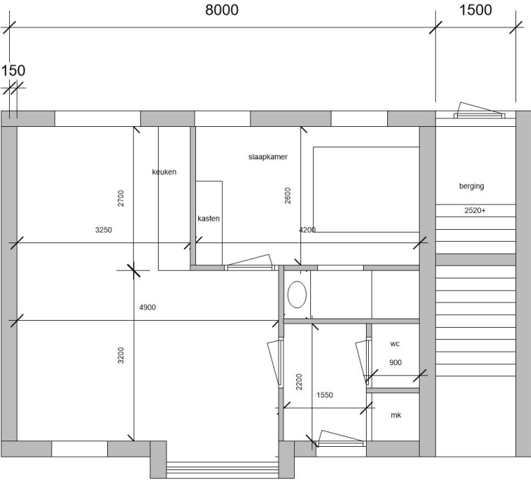
ALTERNATIEF TUSSENWONING BG
