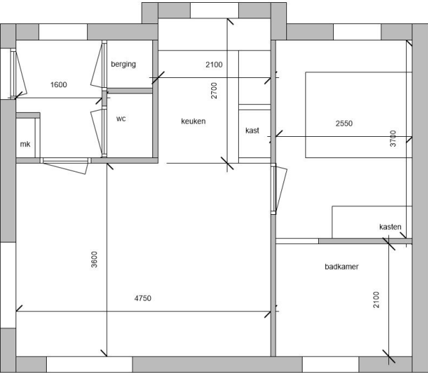
ALTERNATIEF kopwoning Westerweg bg
