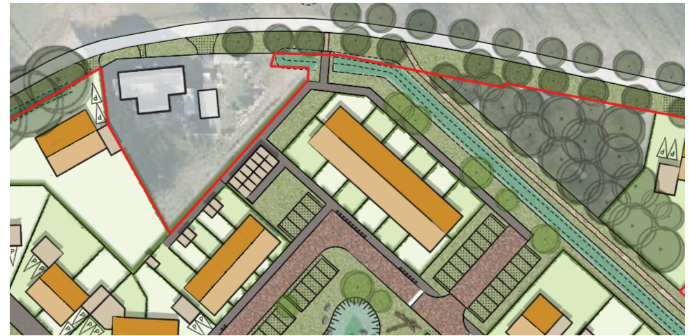
Stedenbouwkundig plan ingezoomd op rug-aan-rugwoningen
