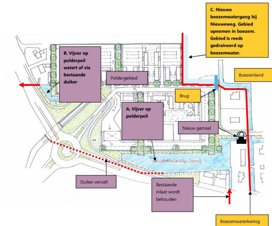
Figuur 4.1: Toekomstig watersysteem
