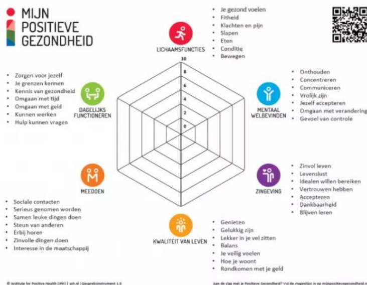
FIGUUR 1 DE ZES DIMENSIES VAN POSITIEVE GEZONDHEID
