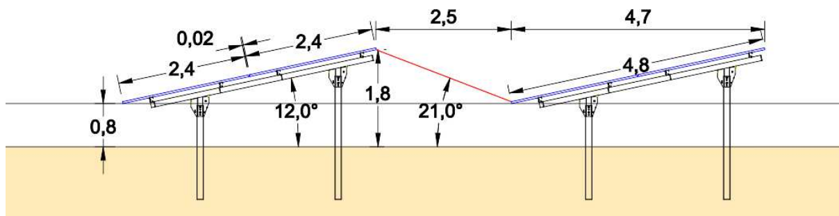
FIGUUR 5: UITSNEDE TECHNISCHE TEKENING VAN DE TE BOUWEN OPSTELLING VAN ZONNEPARK HOOGWOUD. HELE BOUWTEKENING IN BIJLAGE E.
