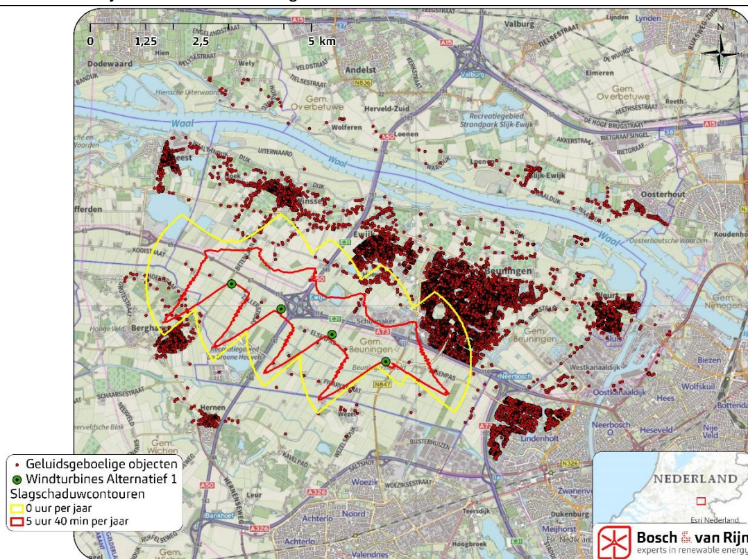
Figuur 6 5:40u en 0:00u slagschaduwcontouren van de alternatieven (volgorde: alternatief 1, alternatief 2 en alternatief 3). Hierbij zijn ook de gevoelige objecten van derden weergegeven. Dit zijn immers de objecten waarvoor de norm geldt.
