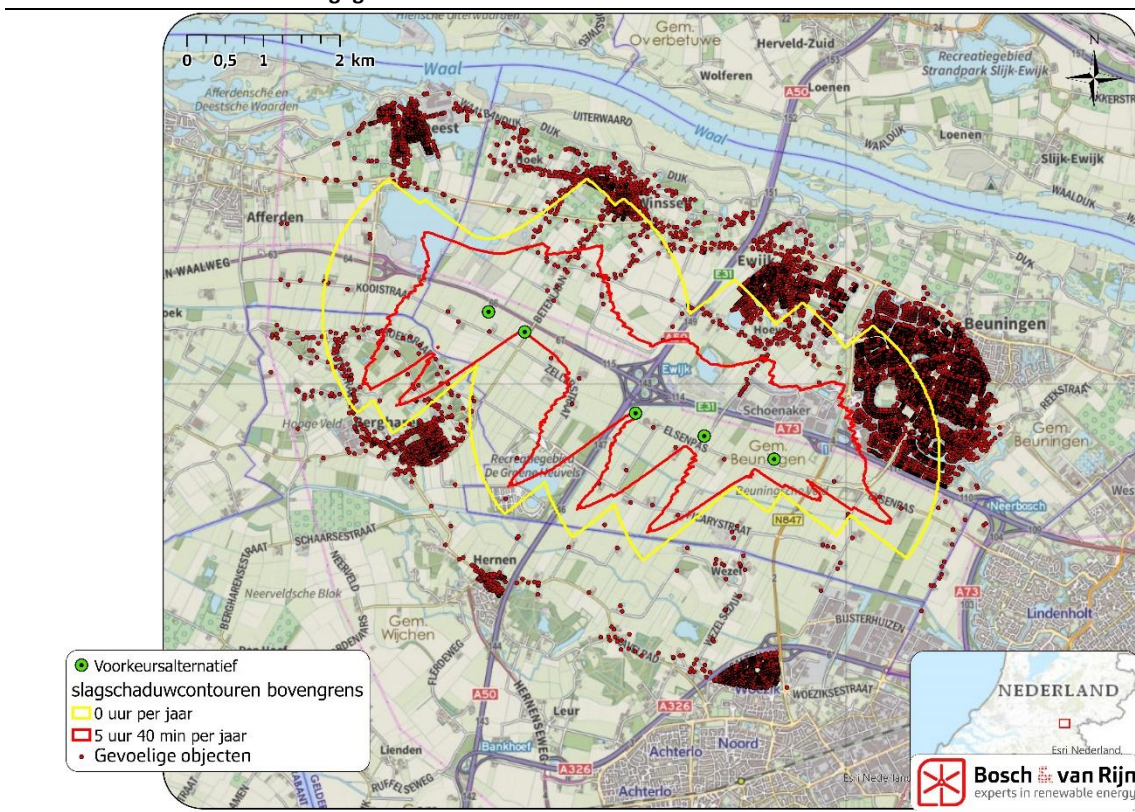
Figuur 9 De 5:40u en 0u slagschaduwcontouren van de bovengrens. Hierbij zijn ook de gevoelige objecten van derden weergegeven.
