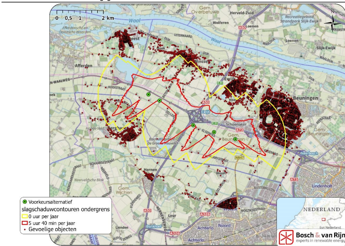
Figuur 8 De 5:40u en 0u slagschaduwcontouren van de ondergrens. Hierbij zijn ook de gevoelige objecten van derden weergegeven.
