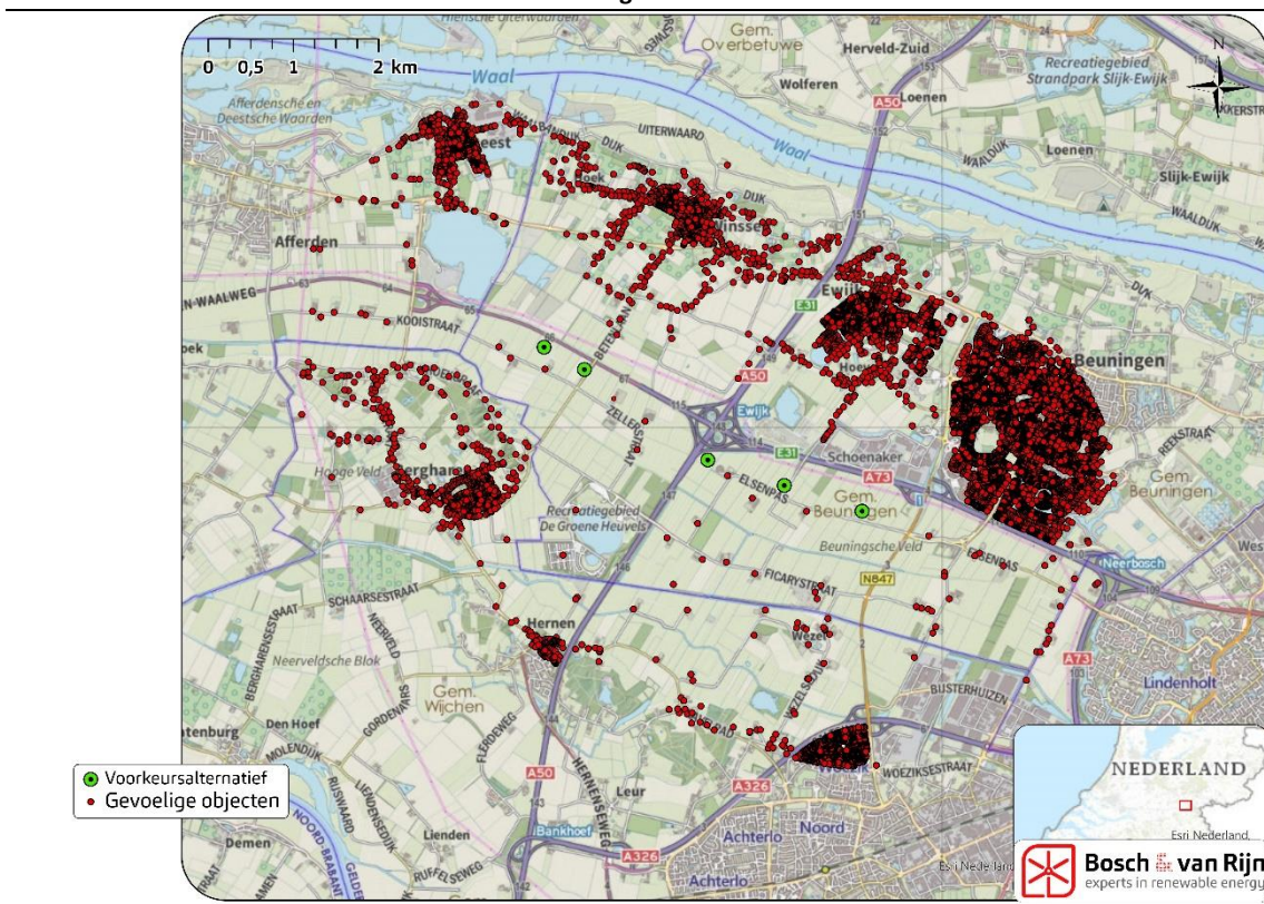
Figuur 7 Windturbinelocaties van het VKA voor windpark Beuningen en alle geluidsgevoelige objecten binnen 12x de rotordiameter van de bovengrens.
