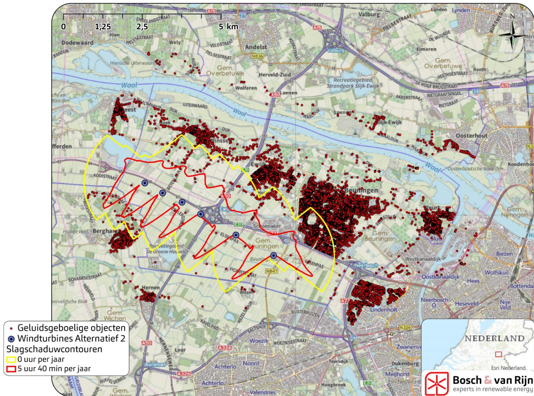
Figuur 11 Slagschaduwcontour Alternatief 2
