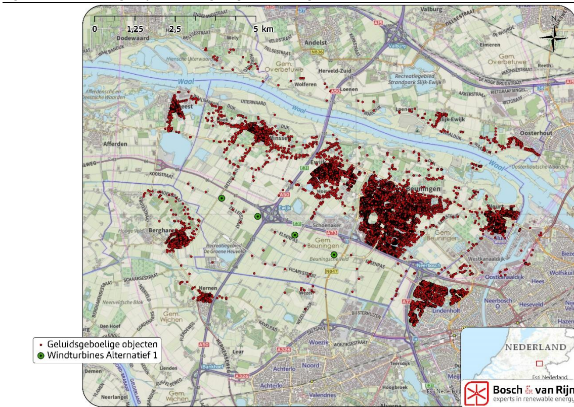
Figuur 4 Gevoelige objecten in omgeving van de beoogde windlocaties.
