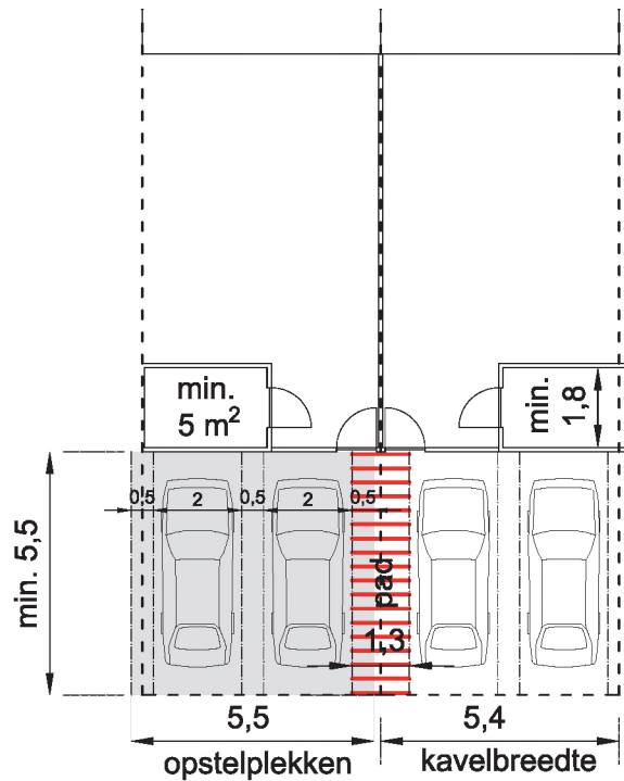
Voorbeelduitwerking opstelplekken en passeerruimte Kavelbreedte 5,40 m. Positie berging achter opstelplekken
