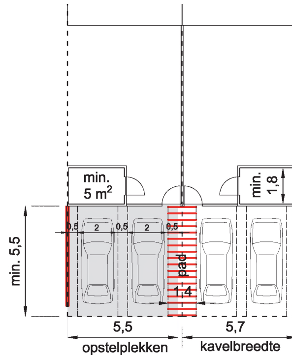
Voorbeelduitwerking opstelplekken en passeerruimte Kavelbreedte 5,70 m. Positie berging achter opstelplekken Vaste erfscheidingsconstructie tussen kavels
