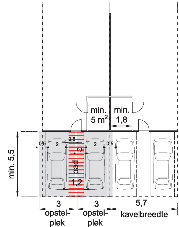
Voorbeelduitwerking opstelplekken en passeerruimte Kavelbreedte 5,70 m. Positie berging achter opstelplekken Passeerruimte per individuele kavel
