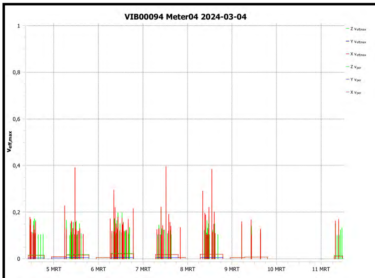
Figuur 7: Trillingen t.g.v. verkeer (inclusief stoortrillingen). Veff,max (dimensieloos getal)
