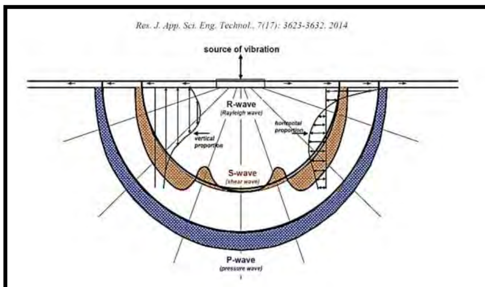
Figuur 3: Diverse trillingsgolven; drukgolf, schuifgolf en Rayleigh golf
