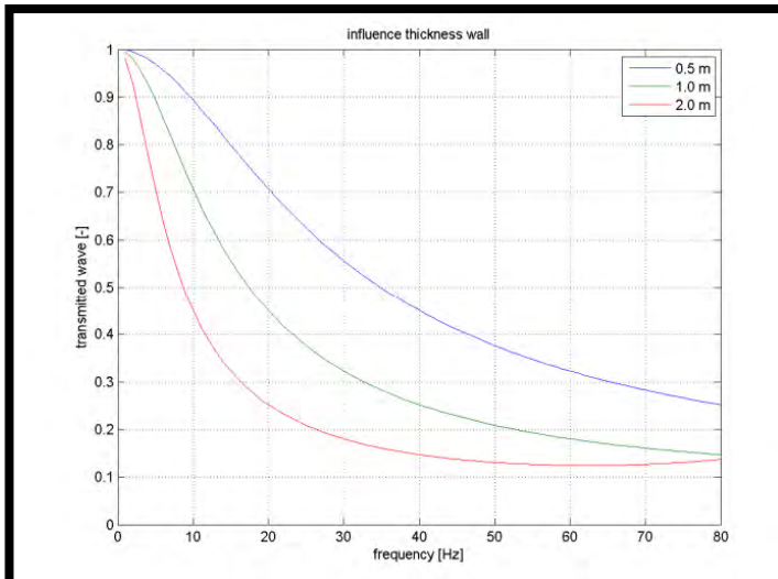
Figuur 14: Invloed dikte van een EPS-scherm in relatie tot het invoegverlies (bron Deltares).
