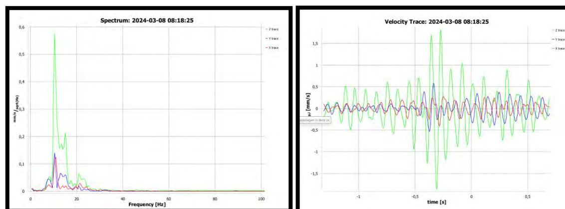
Figuur 6: Hoogst gemeten trilling, links het spectrum en rechts de trace
