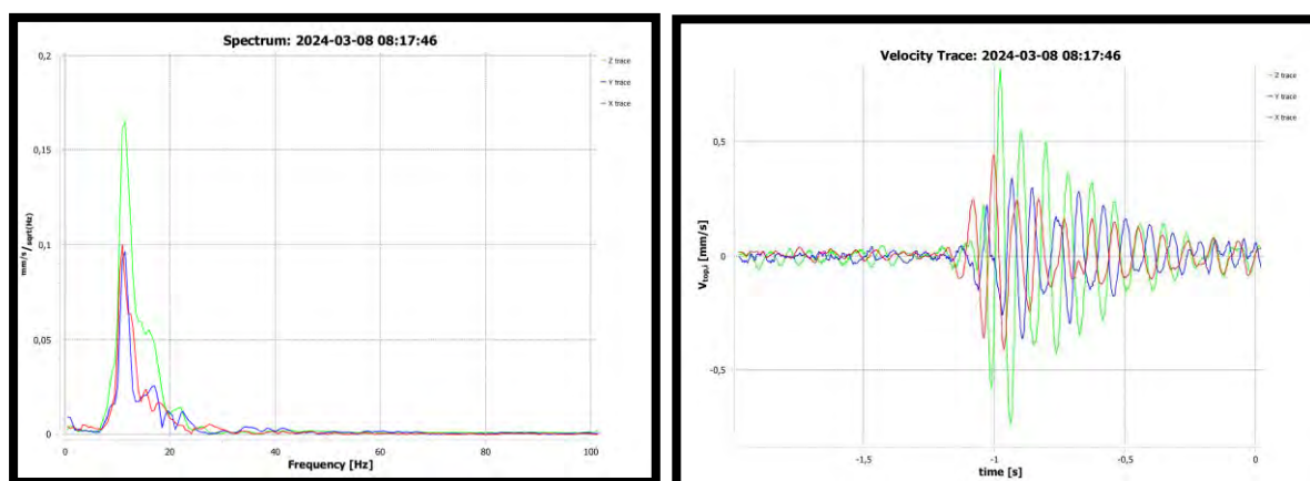
Figuur 10: Hoogst gemeten trilling, links het spectrum en rechts de trace
