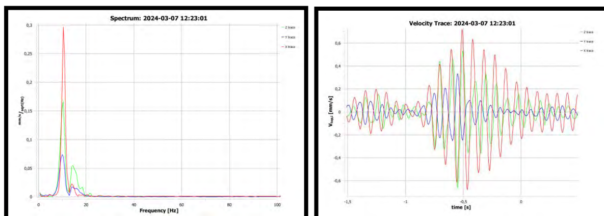
Figuur 8: Hoogst gemeten trilling, links het spectrum en rechts de trace
