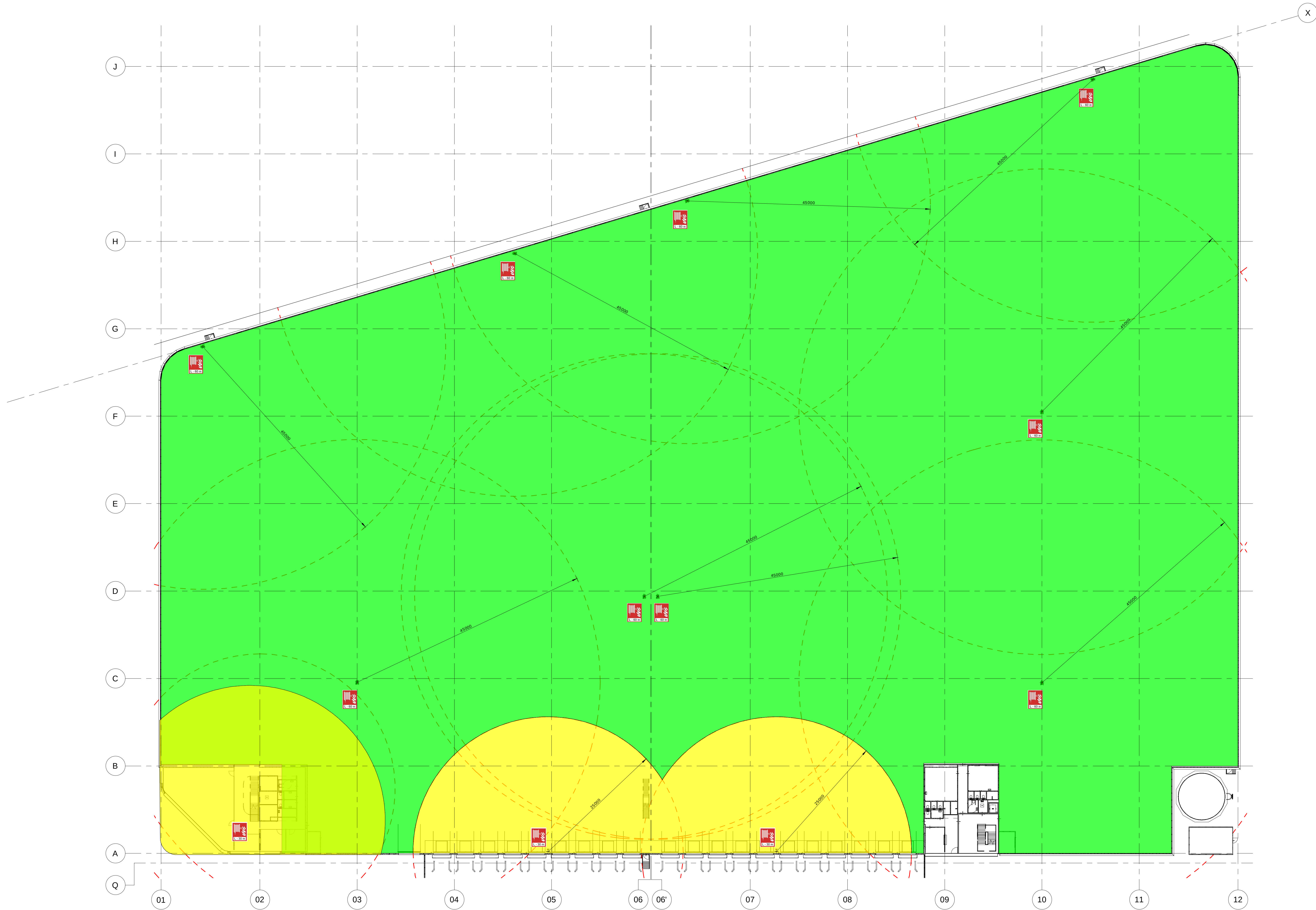
901 Bereik haspelwagens begane grond schaal: 1 : 300
