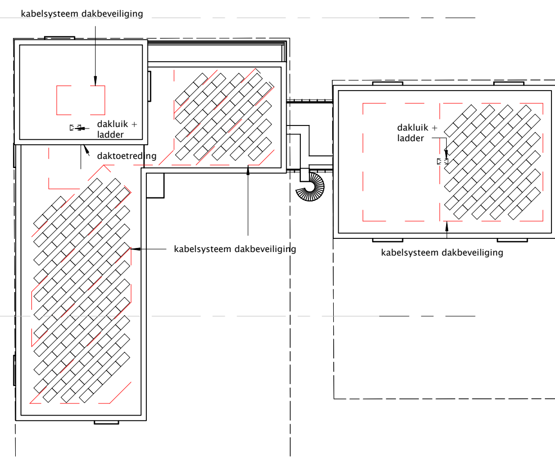
Dakbeveiliging en toetreding 1 : 500
