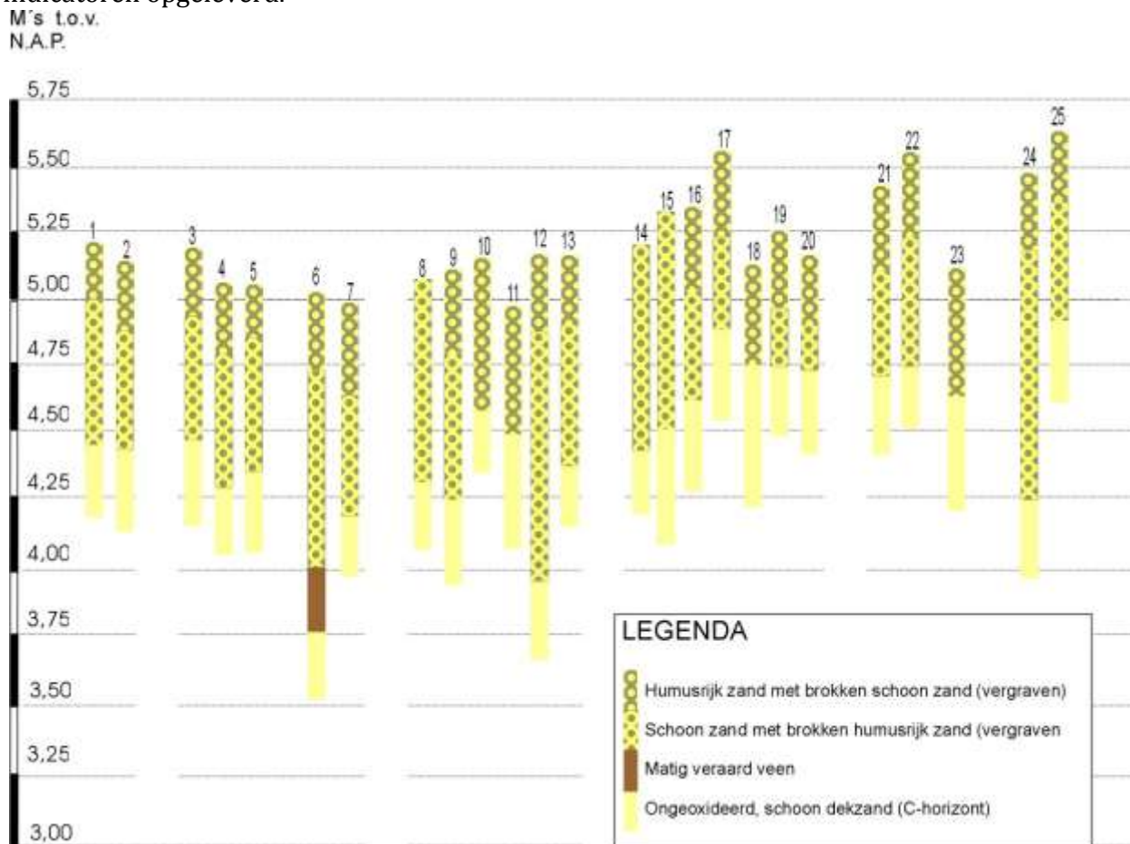
Figuur 20: Boorprofielen
